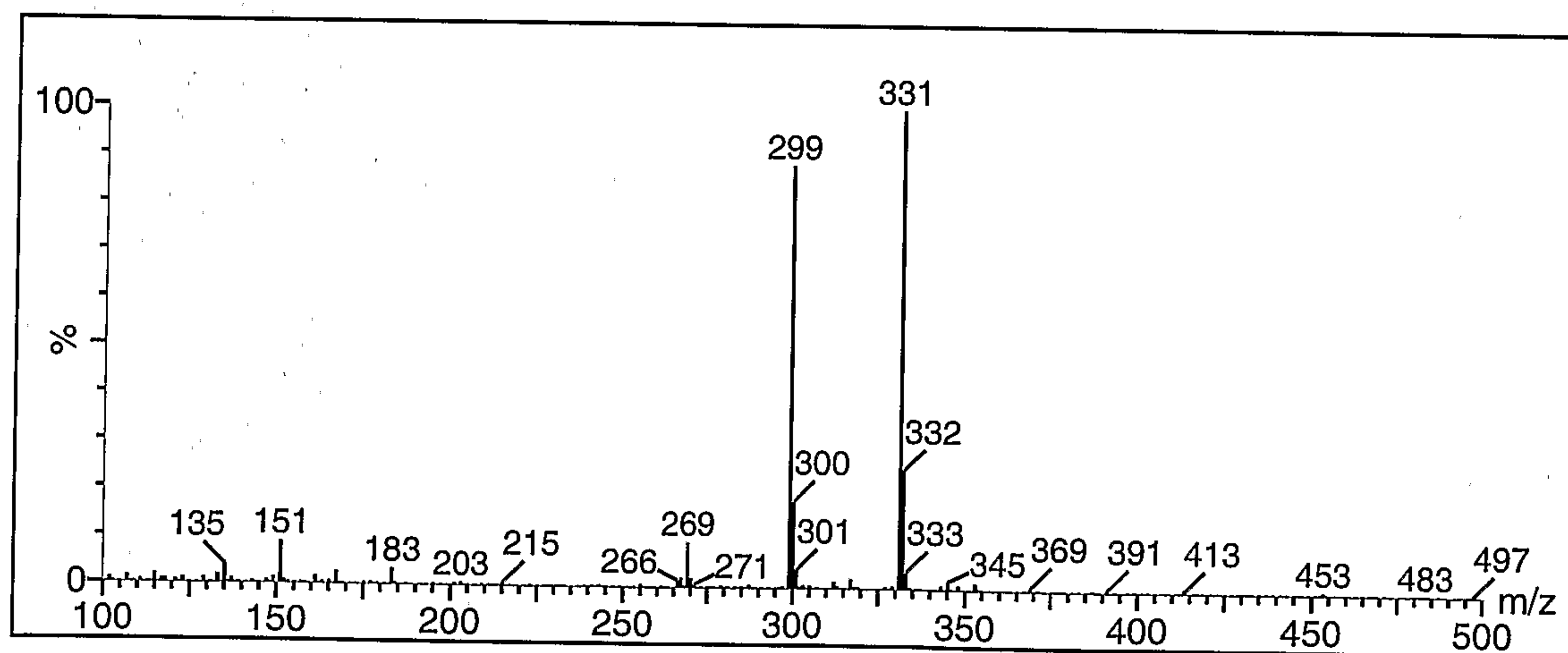
Spectrum - MOM-protected S-equol
