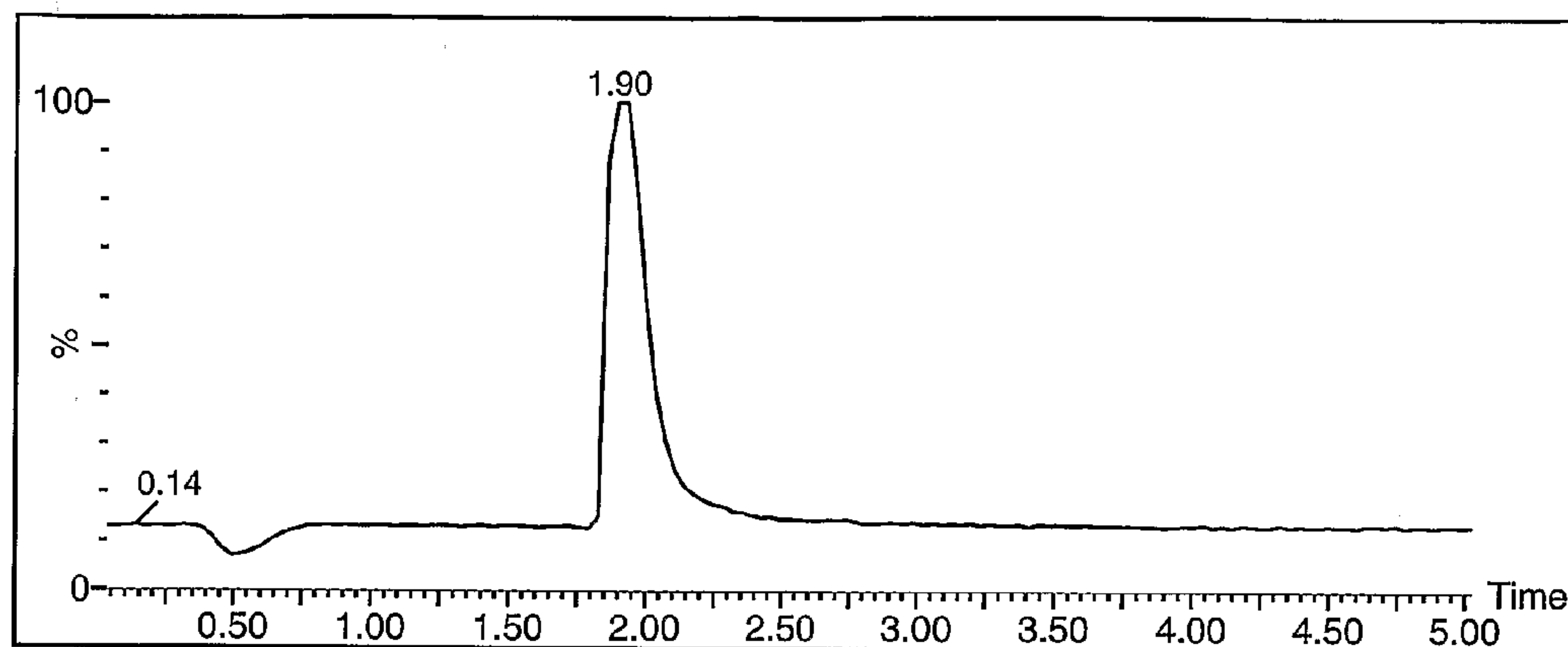
LC Trace - S-Equol
