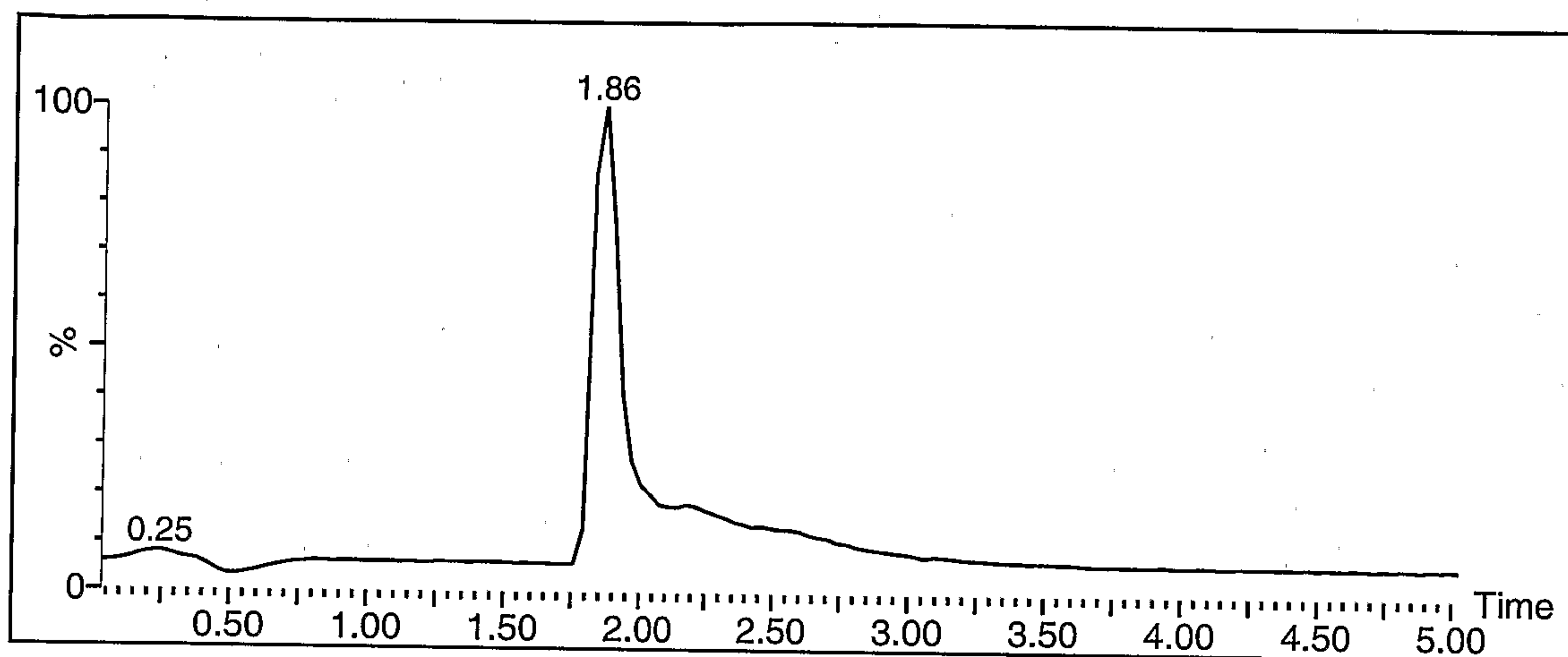
LC Trace - MOM-protected S-equol
