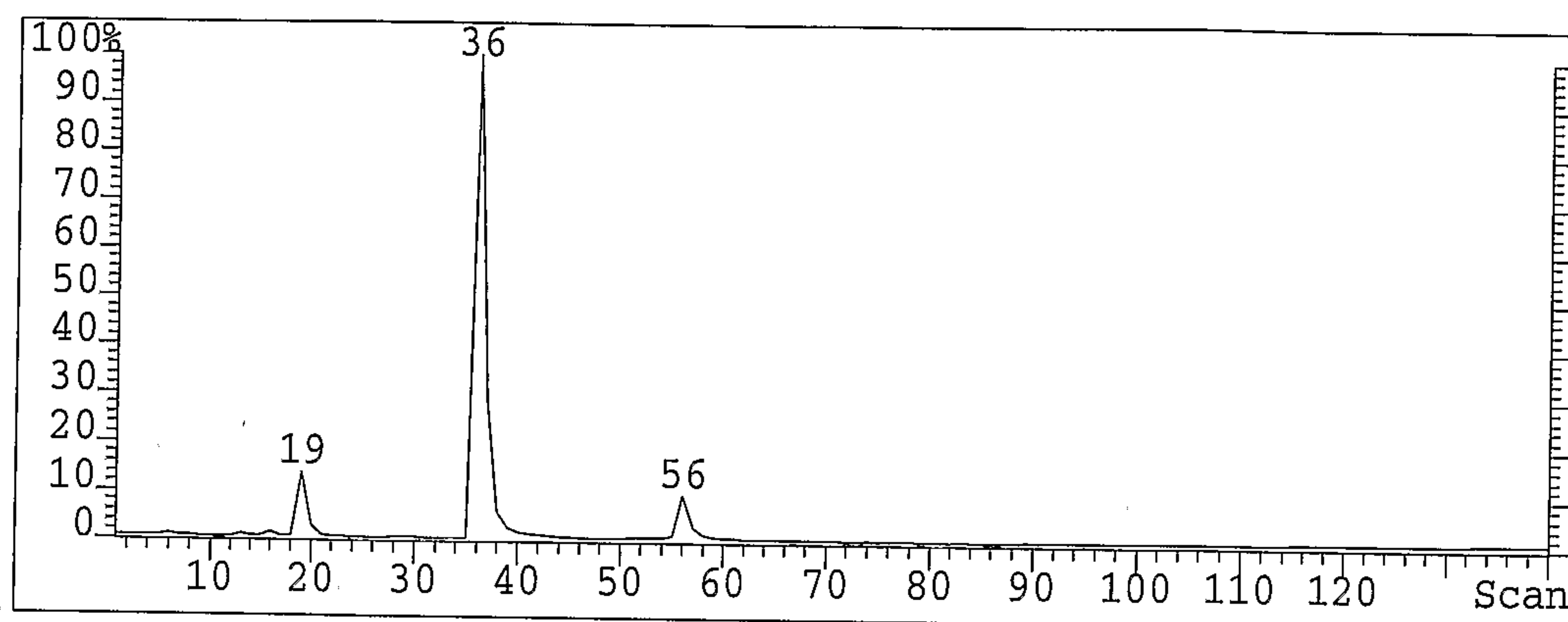
GC Trace - MOM-protected R-equol
