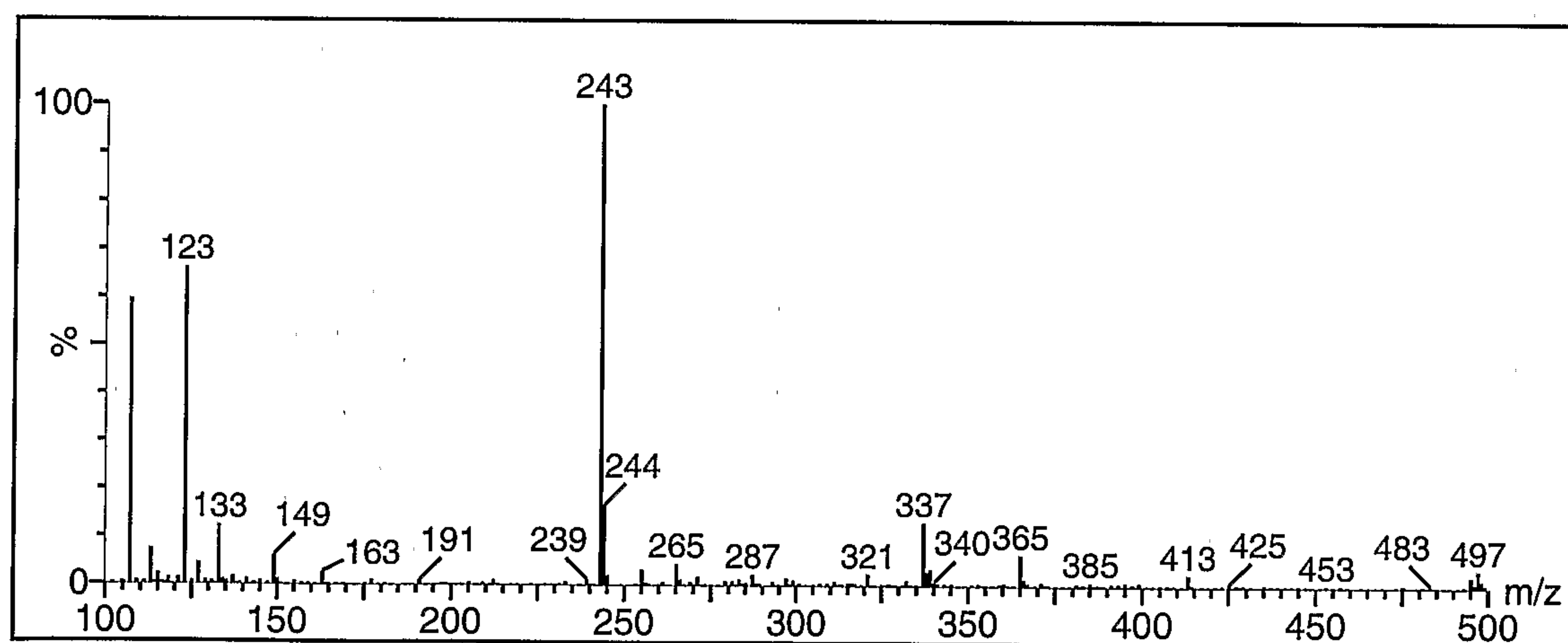
Spectrum - S-Equol
