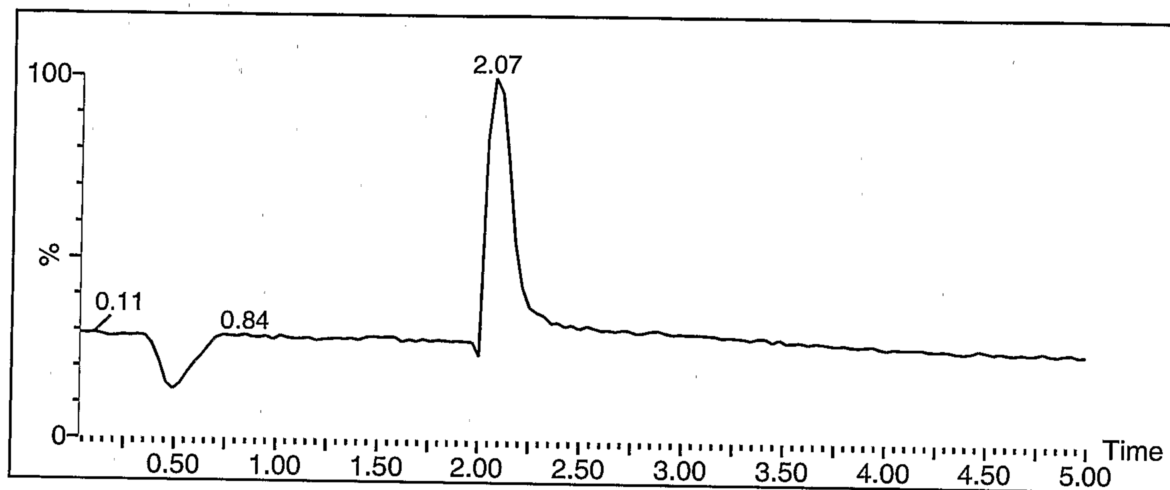
LC Trace - R-Equol
