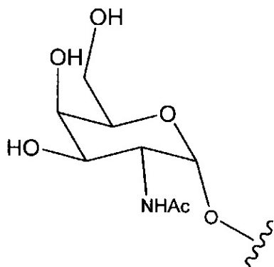
2-(Ацетиламино)-2-дезоксi-α-D-галактопираноза
