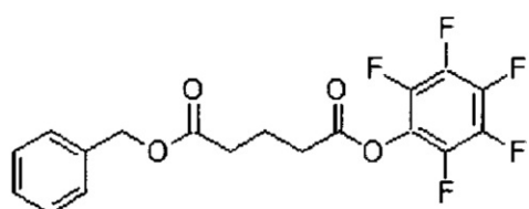
бензил(перфторфенил)тутарат
