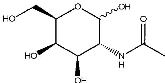
2-(Ацетиламино)-2-дезоксид-D-галактопираноза
