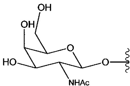
2-(Ацетиламино)-2-дезоксi-β-D-галактопираноза
