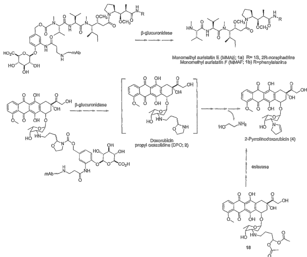
Scheme 2a
