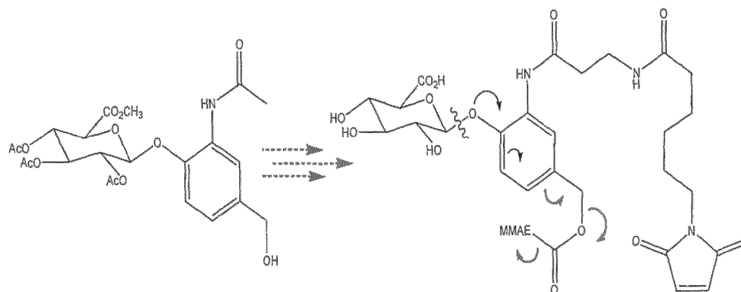
Scheme 2a
