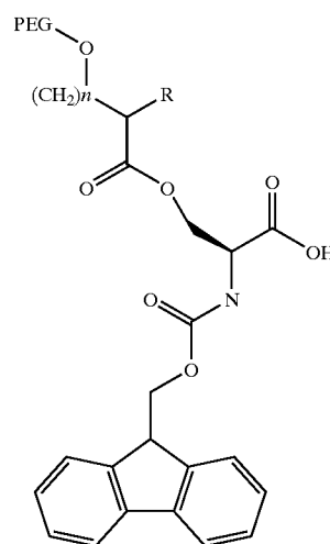
Fmoc-Ser(PEG)-OH
