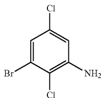
3-bromo-2,5-dichloroaniline
