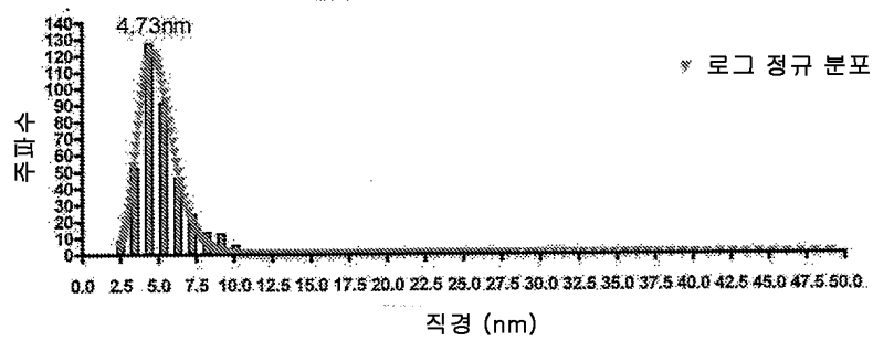
유토피아 골드 TEM 크기 분포
