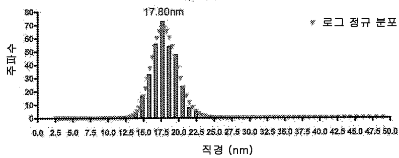
나노콤포식스 15nm TEM 크기 분포
