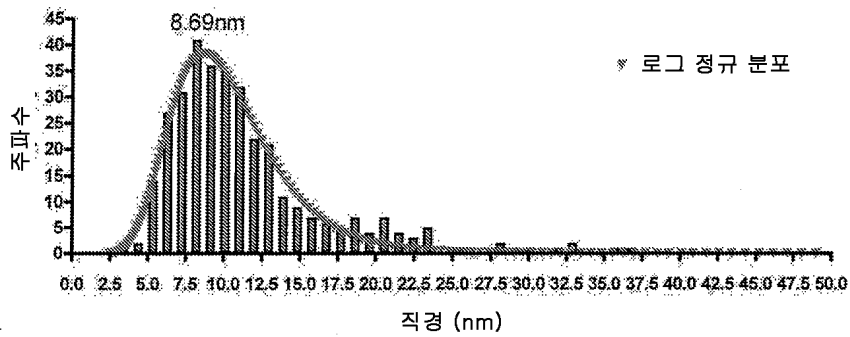
GB-077 TEM 크기 분포
