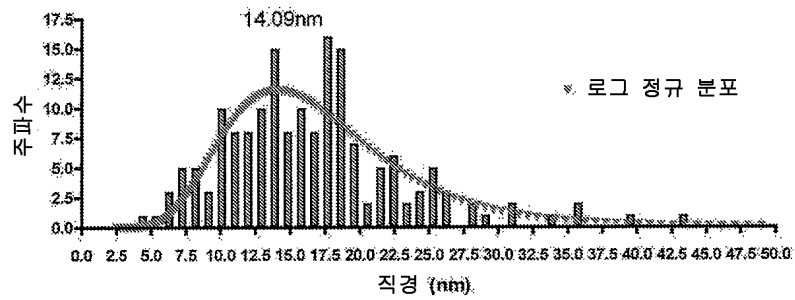
GB-159 TEM크기 분포
