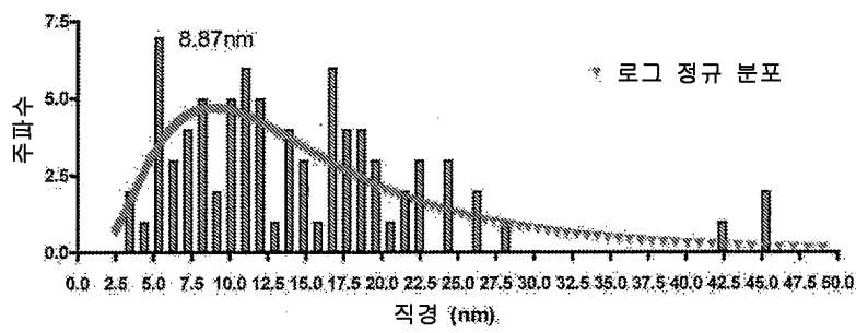
GB-162 TEM크기 분포
