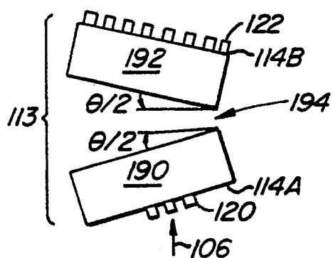
FIG. 15D.
