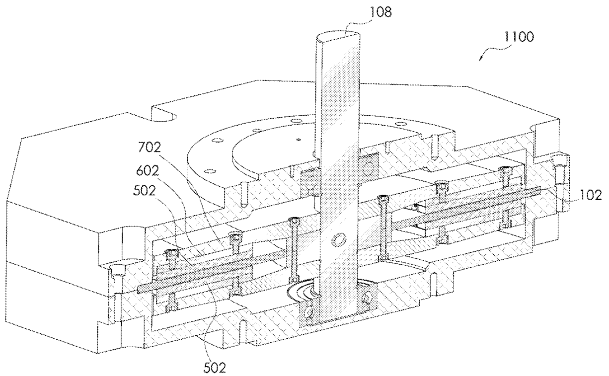
FIG. 11A
