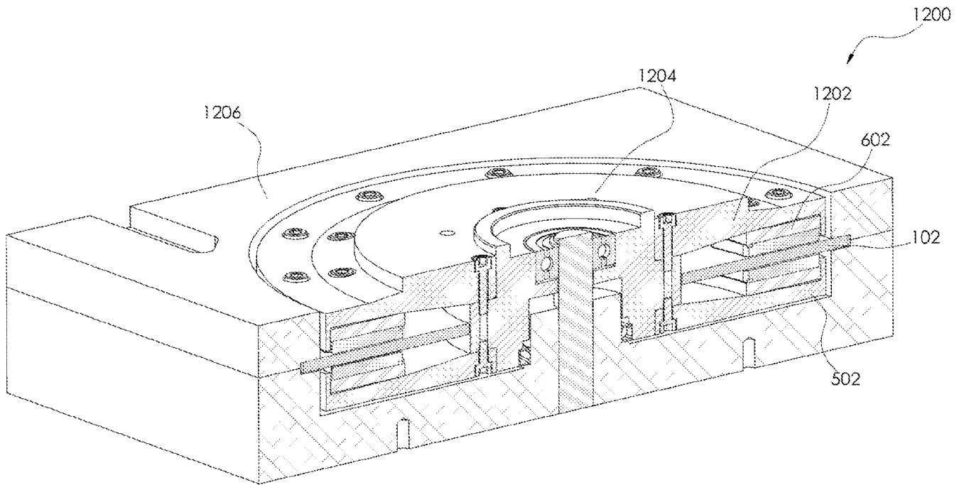
FIG. 12A
