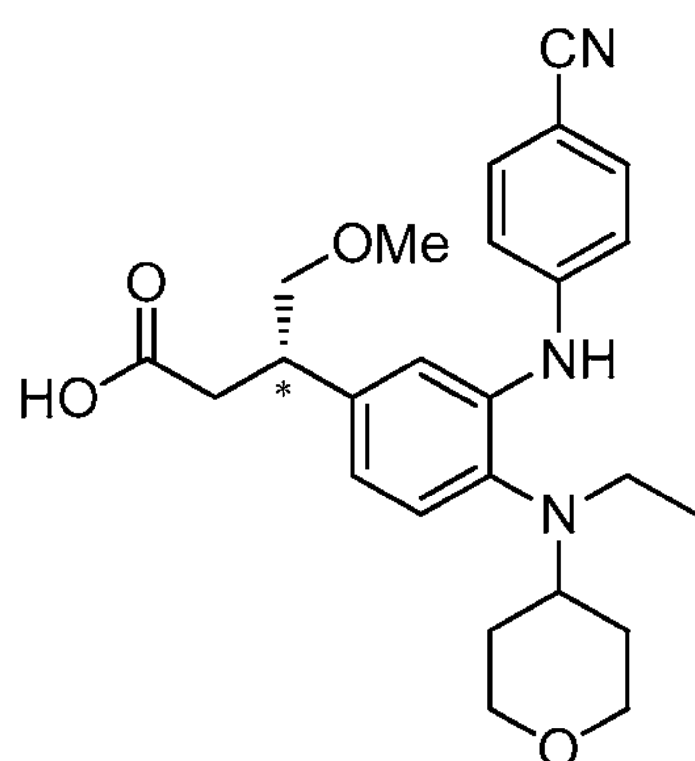
Enantiomer 1
