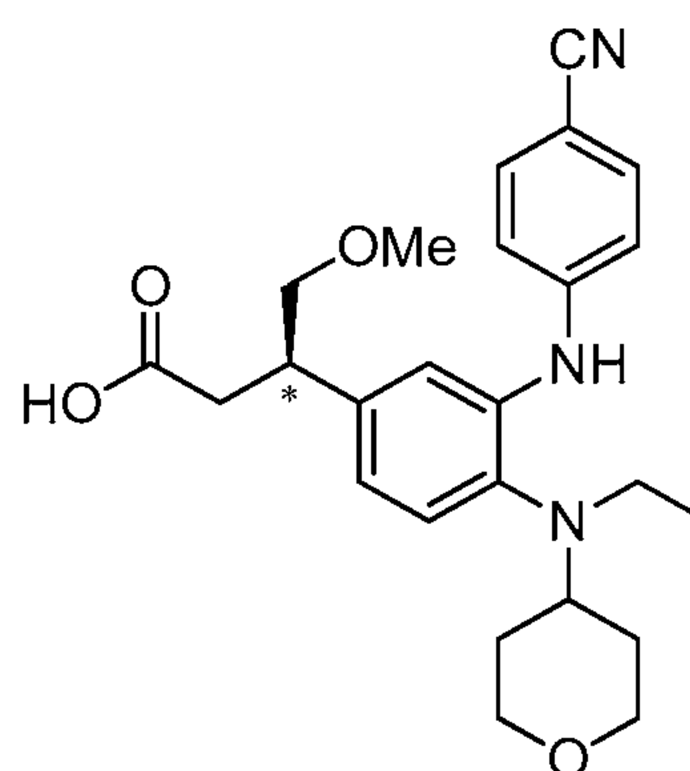
Enantiomer 2
