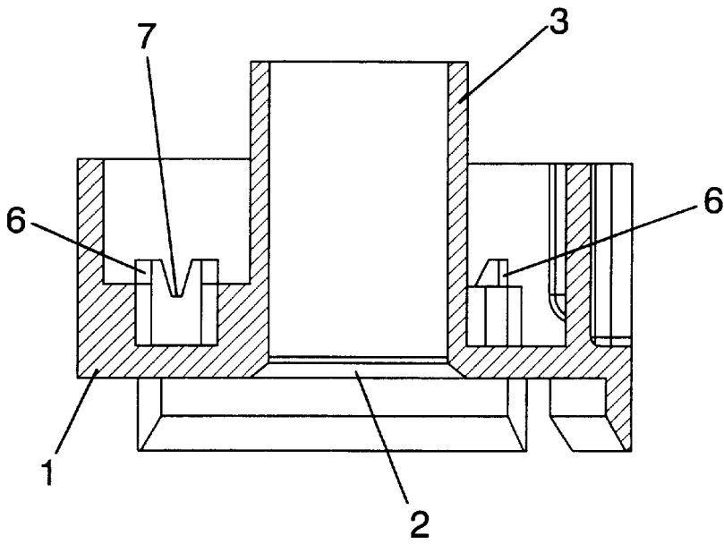
Fig. 3 A-A
