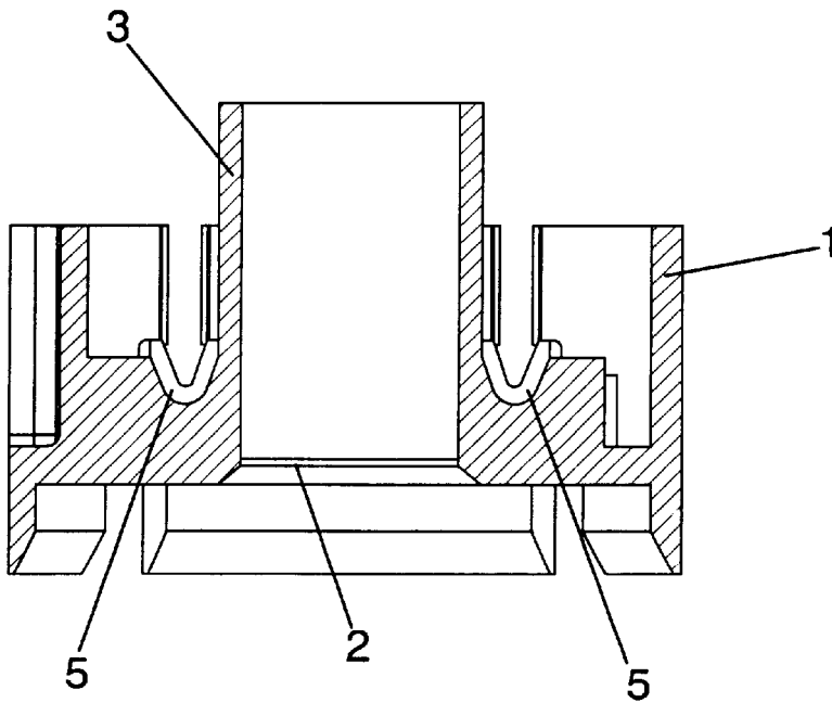
Fig. 4 B-B
