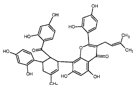
Kuwanon G
