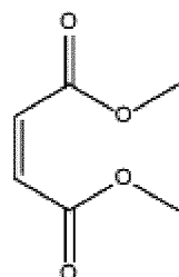
Diethyl maleate ( DEM )
