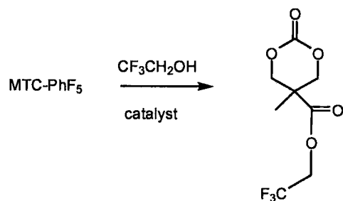
MTC-TFE, (22)
