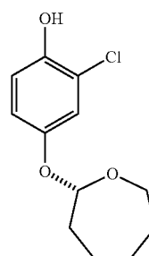
(5)-2-chloro-4-(oxepan-2- yloxy)phenol
