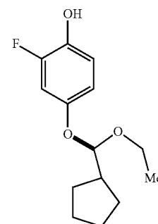
(R)-4-(cyclopentyl(ethoxy)methoxy)-2-fluorophenol
