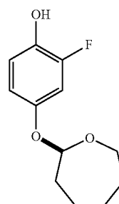
(R)-2-fluoro-4-(oxepan-2- yloxy)phenol
