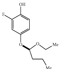
(R)-4-(1-ethoxybutoxy)-2-fluorophenol
