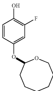
(R)-2-fluoro-4-(oxocan-2-yloxy)phenol
