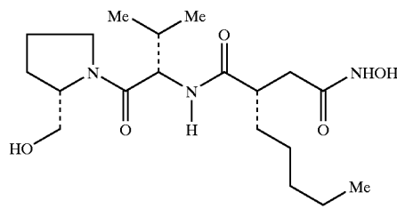
Epiactinonin
