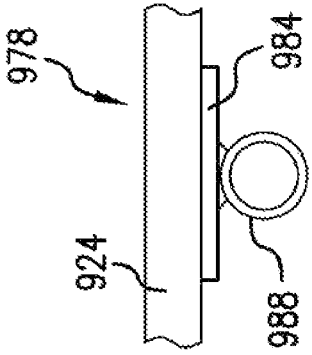
FIG. 15A
