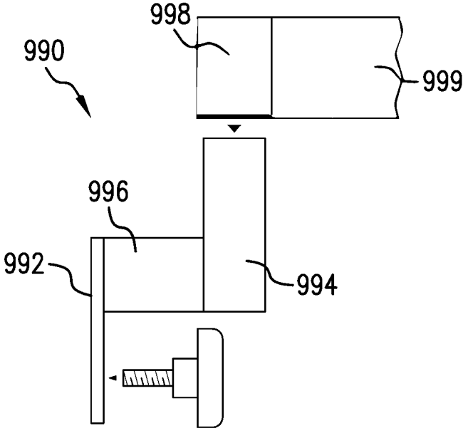
FIG. 17B
