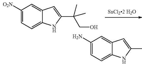
2-(5-Amino-1H-indol-2-yl)-2-methylpropan-1-ol
