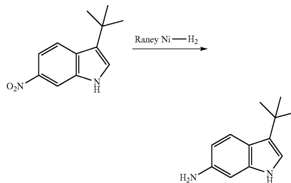
3-tert-Butyl-1H-indol-6-amine
