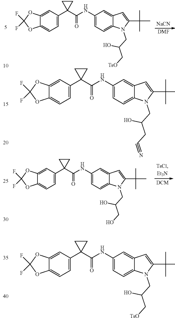
N-(1-(2-Acetamidoethyl)-2-tert-butyl-1H-indol-5-yl)-1-(benzo[d][1,3]-dioxol-5-yl)cyclopropanecarboxamide
