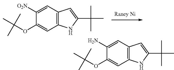
6-tert-Butoxy-2-tert-butyl-1H-indol-5-amine
