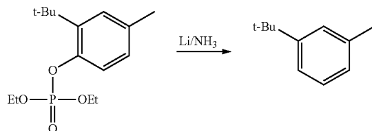
1-tert-Butyl-3-methylbenzene
