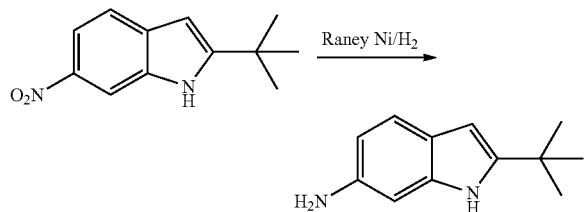
2-tert-Butyl-1H-indol-6-amine
