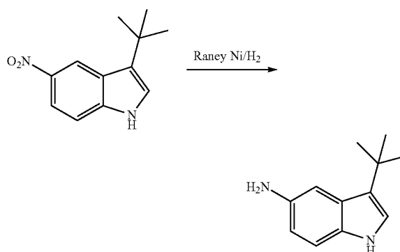
3-tert-Butyl-1H-indol-5-amine
