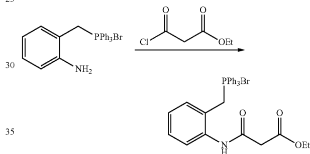
Triphenyl((ethyl(2-carbamoyl)acetate)-2-benzyl)phosphonium bromide
