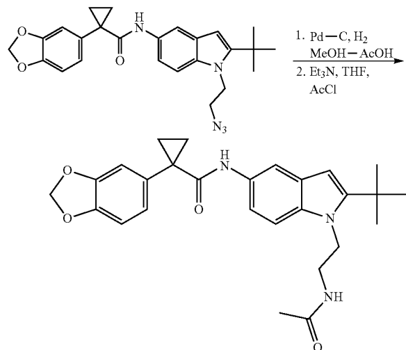
N-(1-(2-Acetamidoethyl)-2-tert-butyl-1H-indol-5-yl)-1-(benzo[d][1,3]-dioxol-5-yl)cyclopropanecarboxamide
