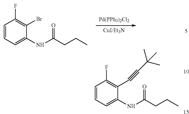
N-(2-(3,3-Dimethylbut-1-ynyl)-3-fluorophenyl)butyramide
