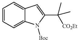
tert-Butyl 2-(2-(ethoxycarbonyl)propan-2-yl)-1H-indole-1-carboxylate
