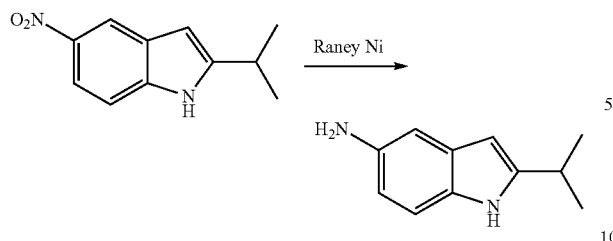
2-Isopropyl-1H-indol-5-amine
