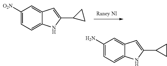
2-Cyclopropyl-1H-indol-5-amine
