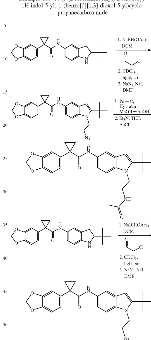
N-(1-(2-azidoethyl)-2-tert-butyl-1H-indol-5-yl)-1-(benzo[d][1,3]dioxol-5-yl)-cyclopropanecarboxamide
