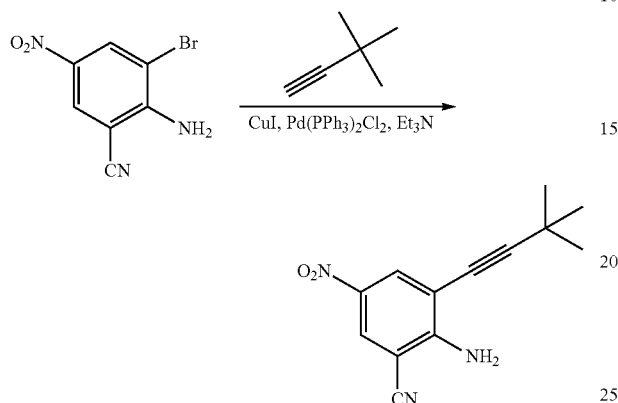
2-Amino-3-(3,3-dimethylbut-1-ynyl)-5-nitrobenzonitrile
