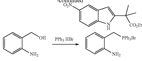
Triphenyl(2-aminobenzyl)phosphonium bromide
