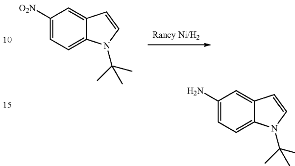
1-tert-Butyl-1H-indol-5-amine
