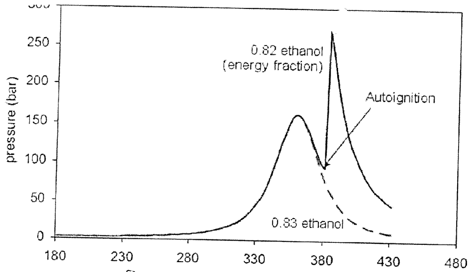
FIG. 2a Crank angle
