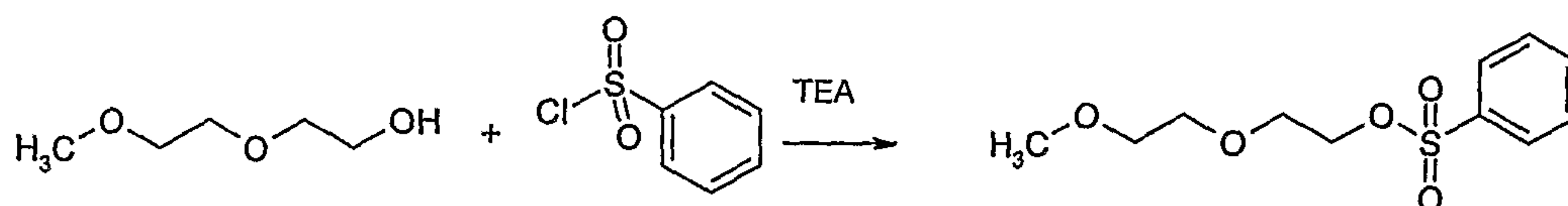
Compound No:83
