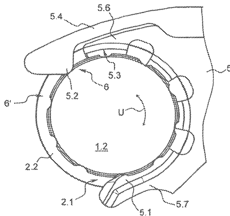
Fig. 5 V-V
