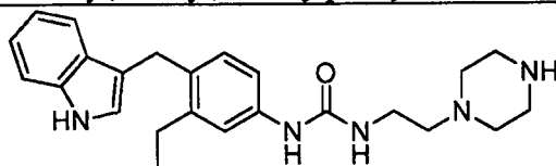
1-(4-((1H-indol-3-yl)methyl)-3-ethylphenyl)-3-(2-(piperazin-1-yl)ethyl)urea;
