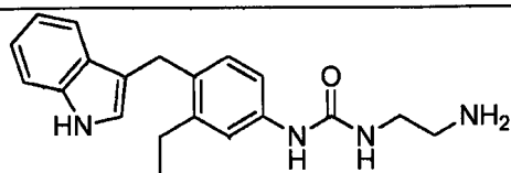
1-(4-((1H-indol-3-yl)methyl)-3-ethylphenyl)-3-(2-aminoethyl)urea;
