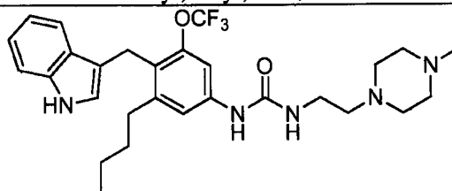
1-(4-((1H-indol-3-yl)methyl)-3-butyl-5-(trifluoromethoxy)phenyl)-3-(2-(4-methylpiperazin-1-yl)ethyl)urea;
