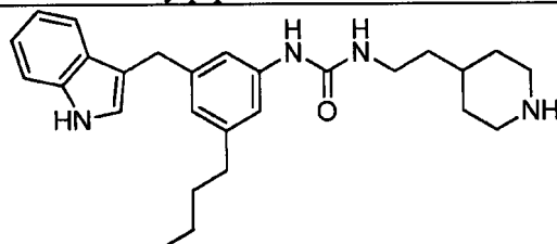
1-(3-((1H-indol-3-yl)methyl)-5-butylphenyl)-3-(2-(piperidin-4-yl)ethyl)urea;
