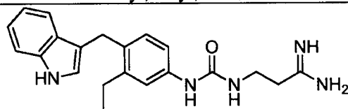
3-(3-(4-((1H-indol-3-yl)methyl)-3-ethylphenyl)ureido)propanimidamide;
