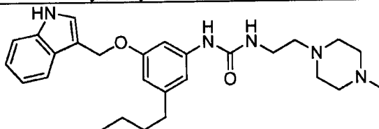
1-(3-((1H-indol-3-yl)methoxy)-5-butylphenyl)-3-(2-(4-methylpiperazin-1-yl)ethyl)urea;
