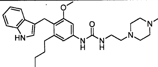
1-(4-((1H-indol-3-yl)methyl)-3-butyl-5-methoxyphenyl)-3-(2-(4-methylpiperazin-1-yl)ethyl)urea;
