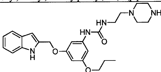
1-(3-((1H-indol-2-yl)methoxy)-5-propoxyphenyl)-3-(2-(piperazin-1-yl)ethyl)urea
