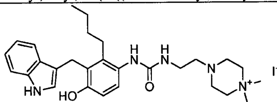
4-(2-(3-(4-((1H-indol-3-yl)methyl)-3-butyl-5-hydroxyphenyl)ureido)ethyl)-1,1-dimethylpiperazin-1-ium iodide;
