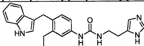
1-(2-(1H-imidazol-5-yl)ethyl)-3-(4-((1H-indol-3-yl)methyl)-3-ethylphenyl)urea;
