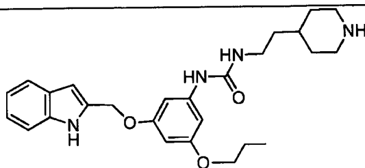
1-(3-((1H-indol-2-yl)methoxy)-5-propoxyphenyl)-3-(2-(piperidin-4-yl)ethyl)urea
