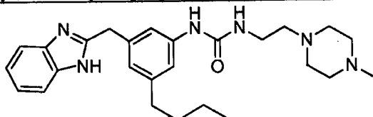
1-(3-((1H-benzo[d]imidazol-2-yl)methyl)-5-butylphenyl)-3-(2-(4-methylpiperazin-1-yl)ethyl)urea
