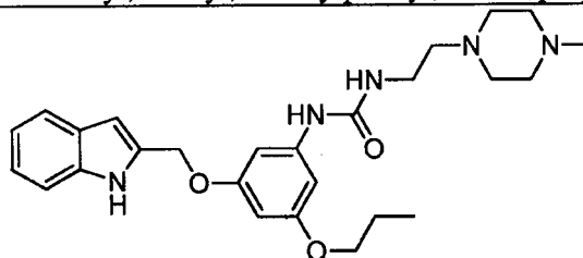
1-(3-((1H-indol-2-yl)methoxy)-5-propoxyphenyl)-3-(2-(4-methylpiperazin-1-yl)ethyl)urea;
