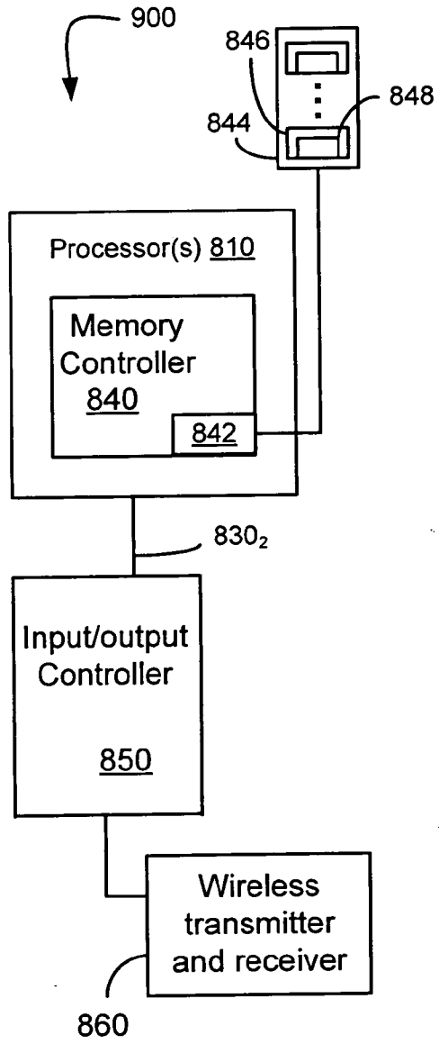
Fig. 8B
