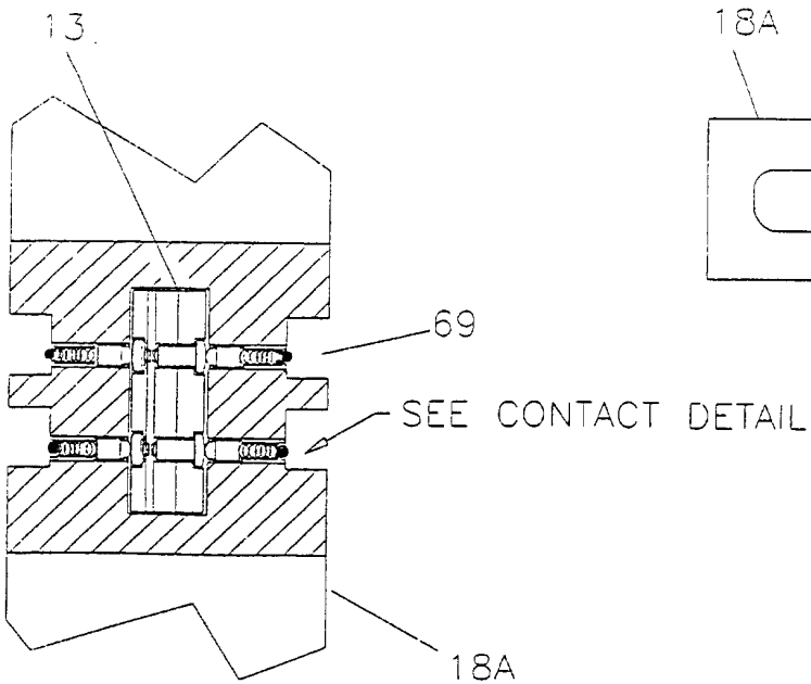
SECTION D-D FIG. 13
