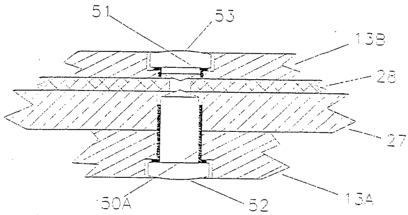
SECTION A-A FIG. 12
