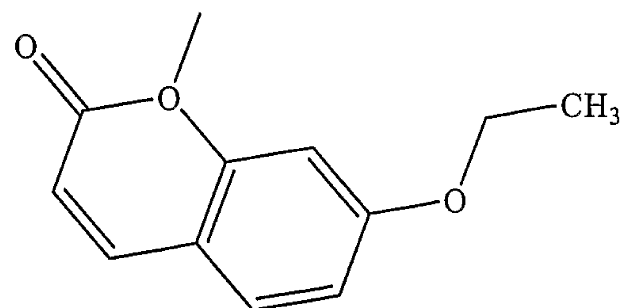
(7-ethoxycoumarin)
