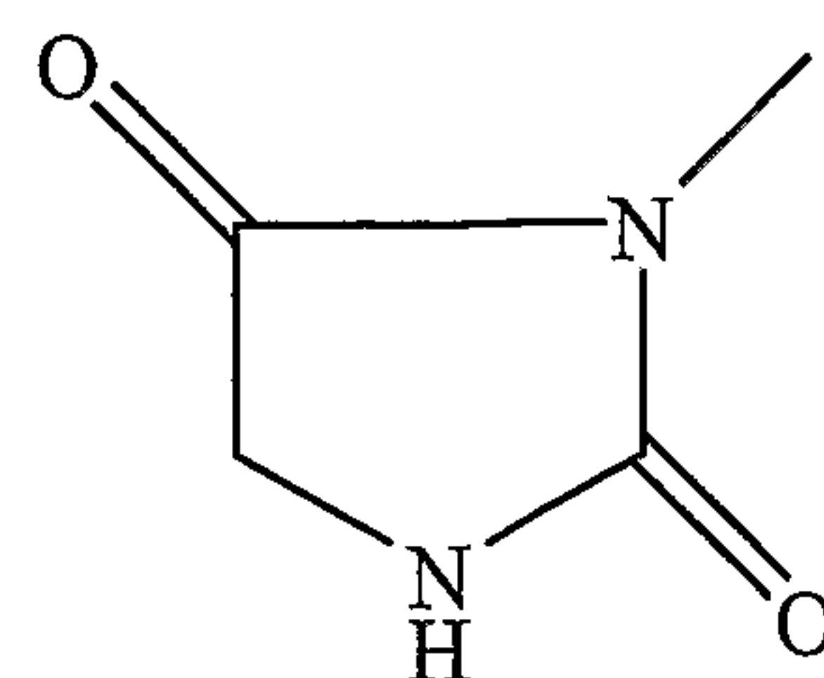
(hydantoin)
