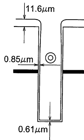
(d) CVD method
