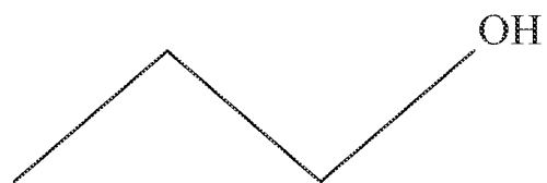
1 - butanol
