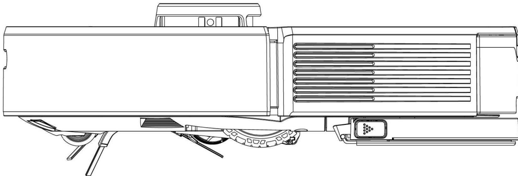
右側視圖
