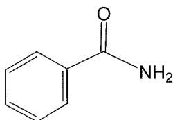
benzamide
