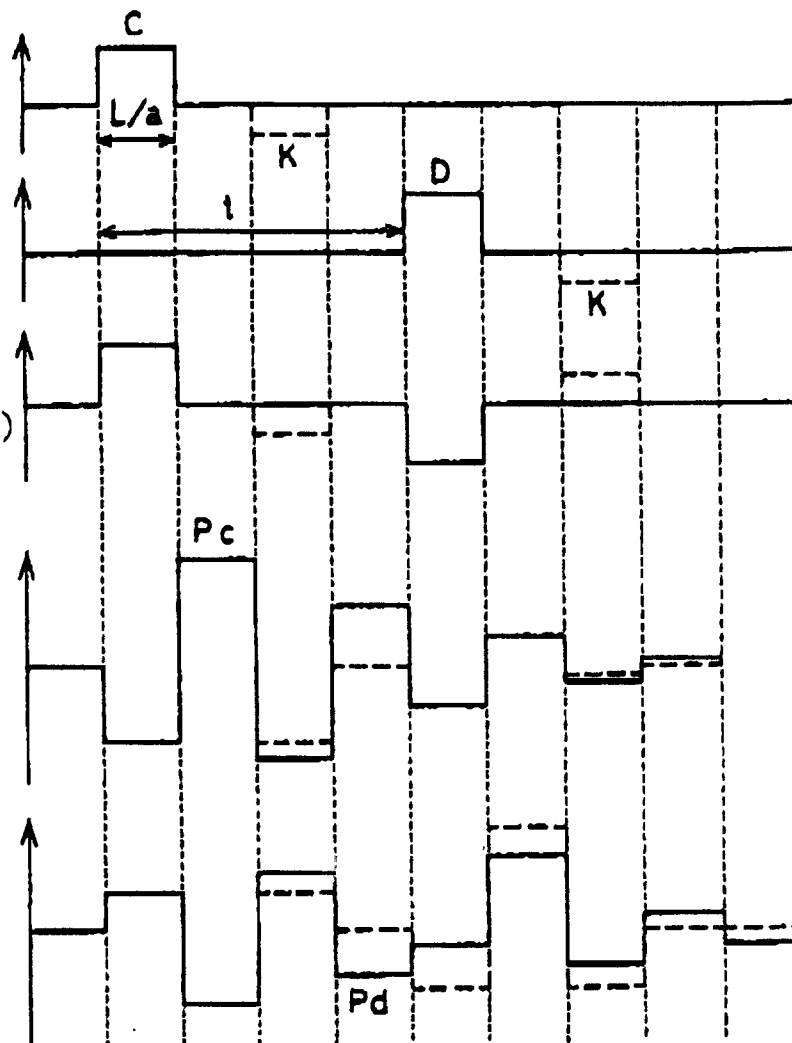
FIG. 6 (d) PRESSURE NEAR NOZZLE (4c)
