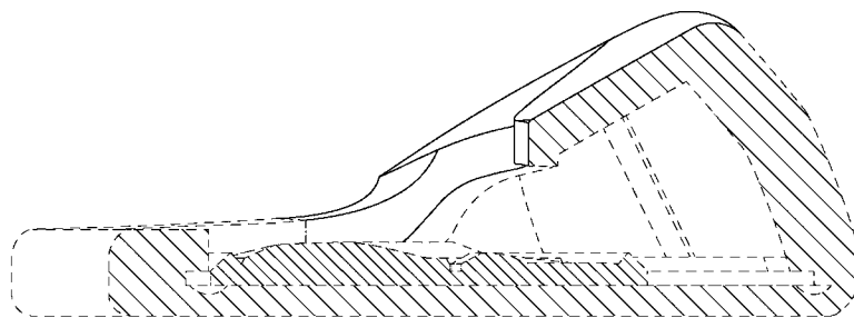
【A-A剖視圖】
