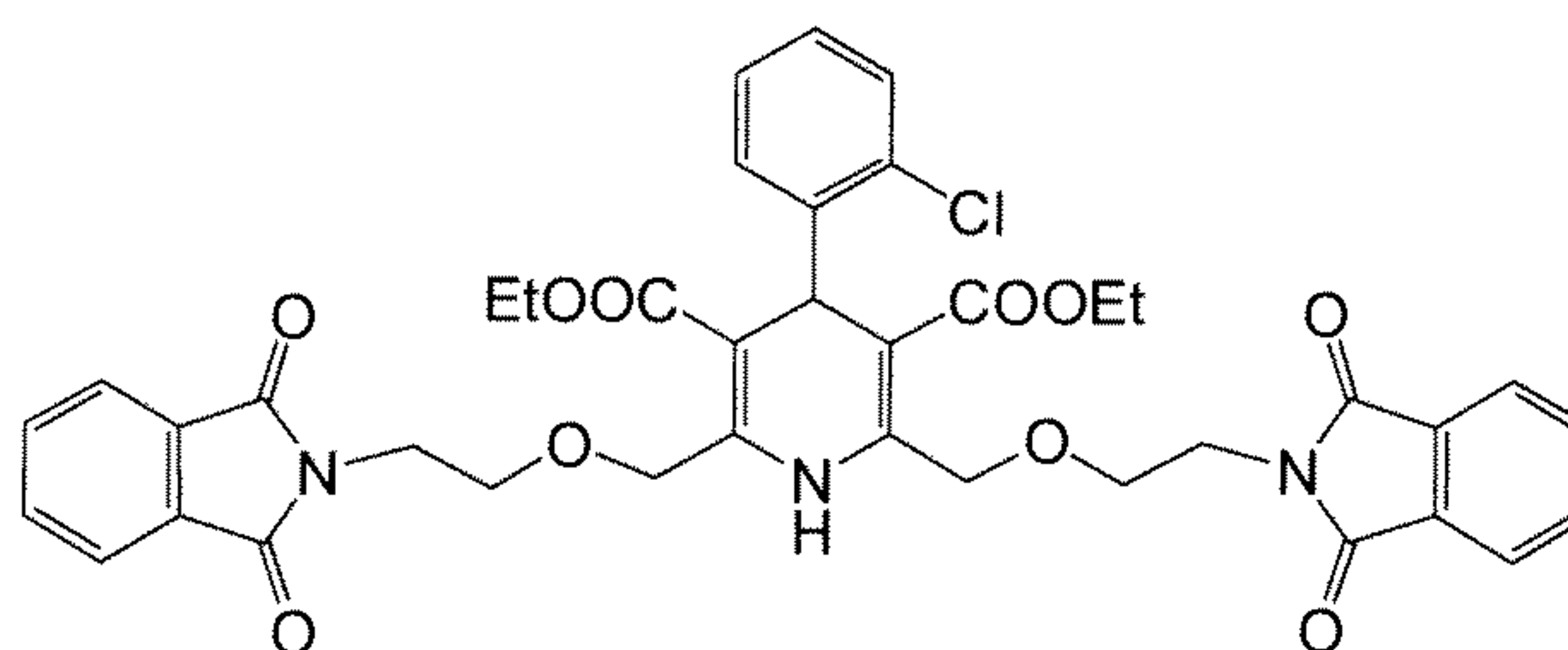
impurity HA
