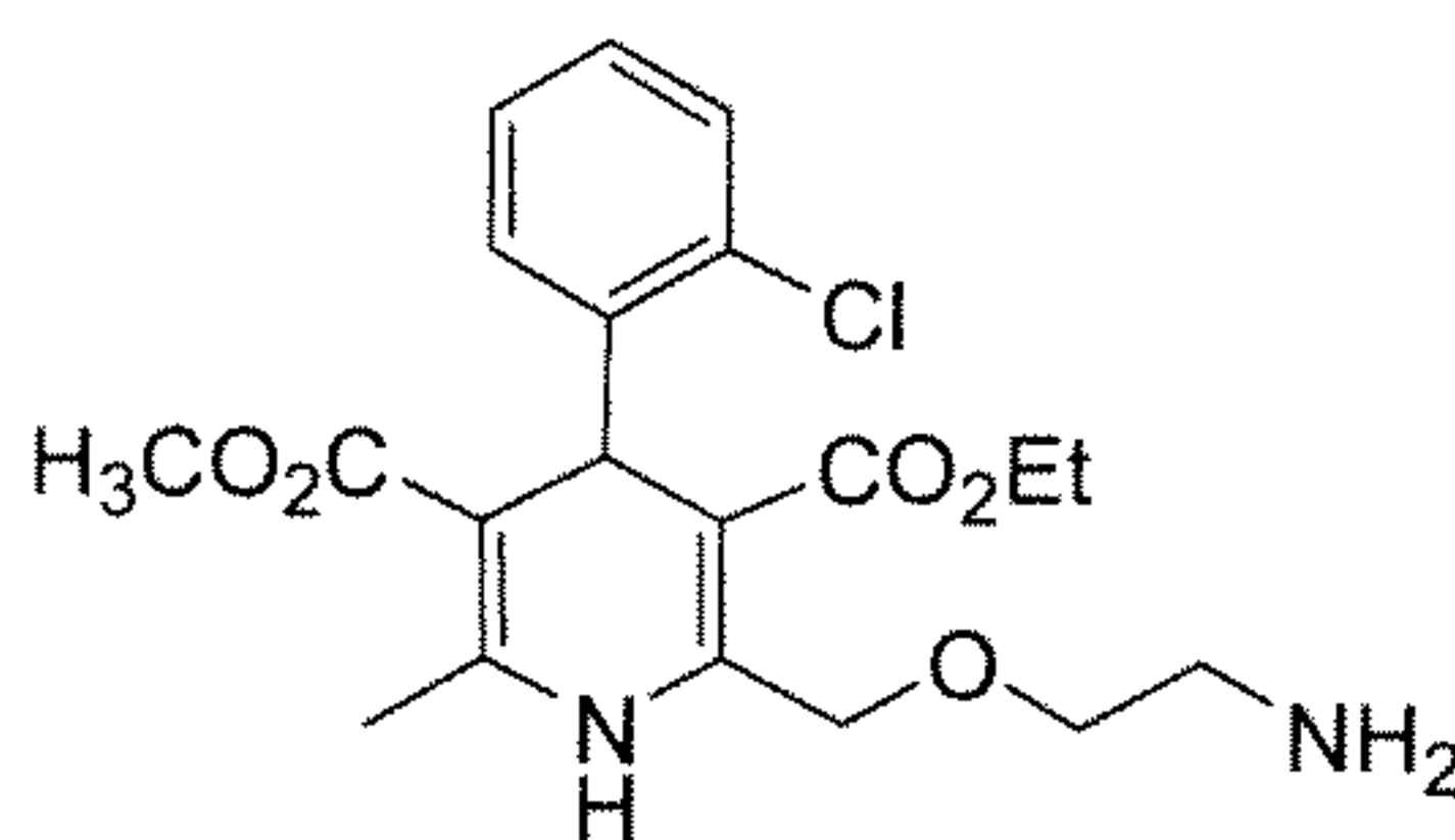
Amlodipine
