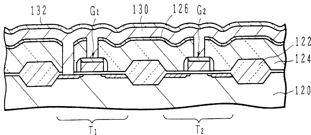
FIG.24
