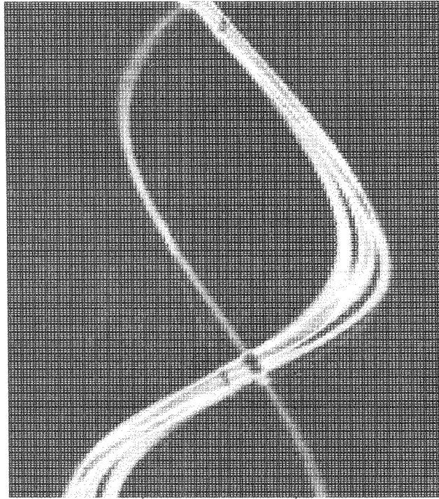
Sinogram M 1204
