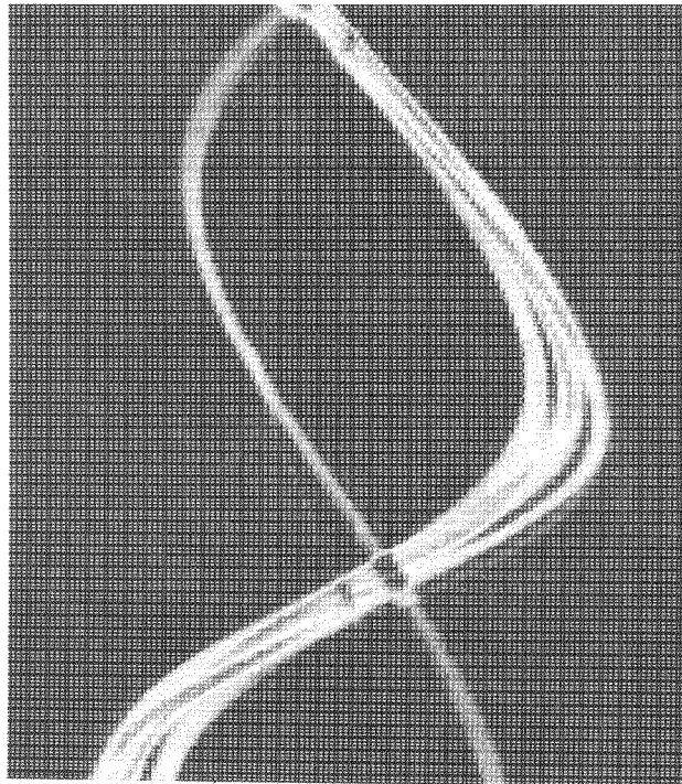
Sinogram P 1206
