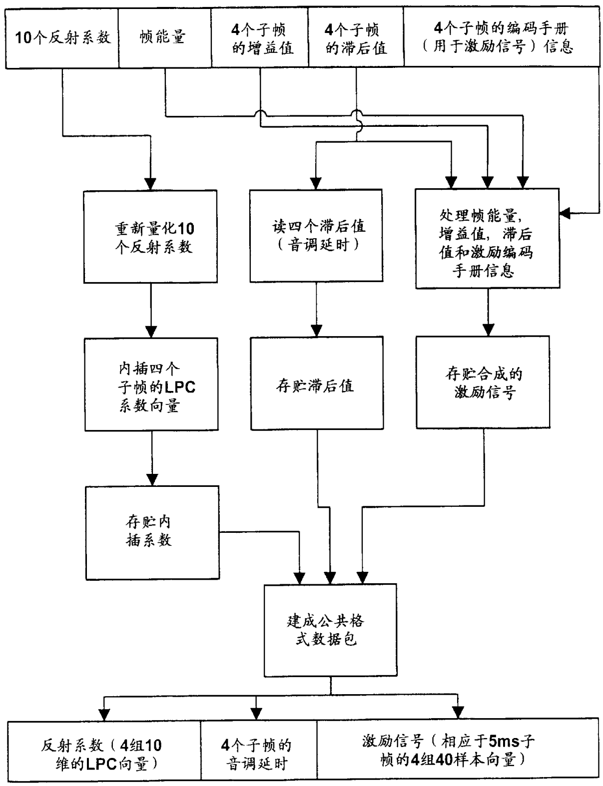
公共格式帧
