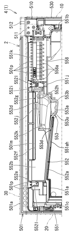
B1-B1断面图
