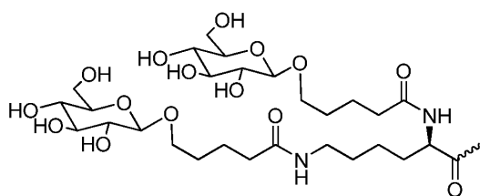
[0439] 화학식 XVIII,
