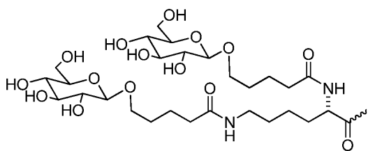
[0438] 화학식 XVII,
