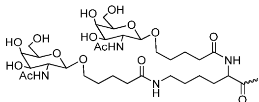
[0437] 화학식 XVI,
