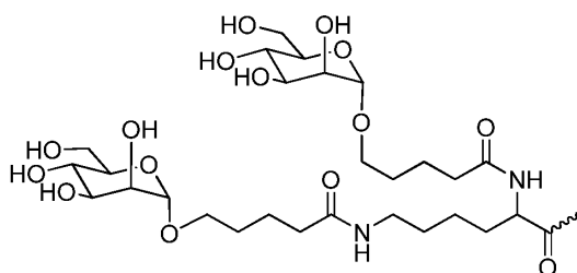
[0441] 화학식 XX,
