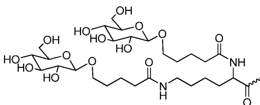
[0440] 화학식 XIX,
