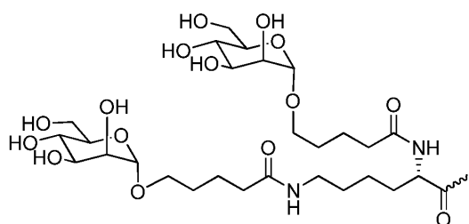
[0442] 화학식 XXI,
