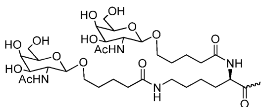
[0436] 화학식 XV,
