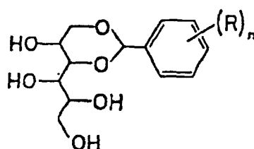
Formule (I-c)
