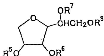
Formule (I-e)
