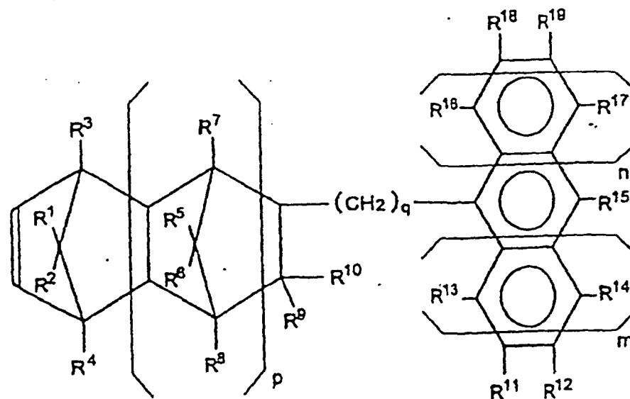
Formule (III)
