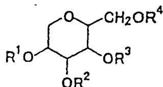
Formule (I-d)
