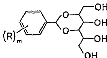
Formule (I-b)
