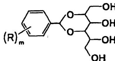
Formula (I-b)
