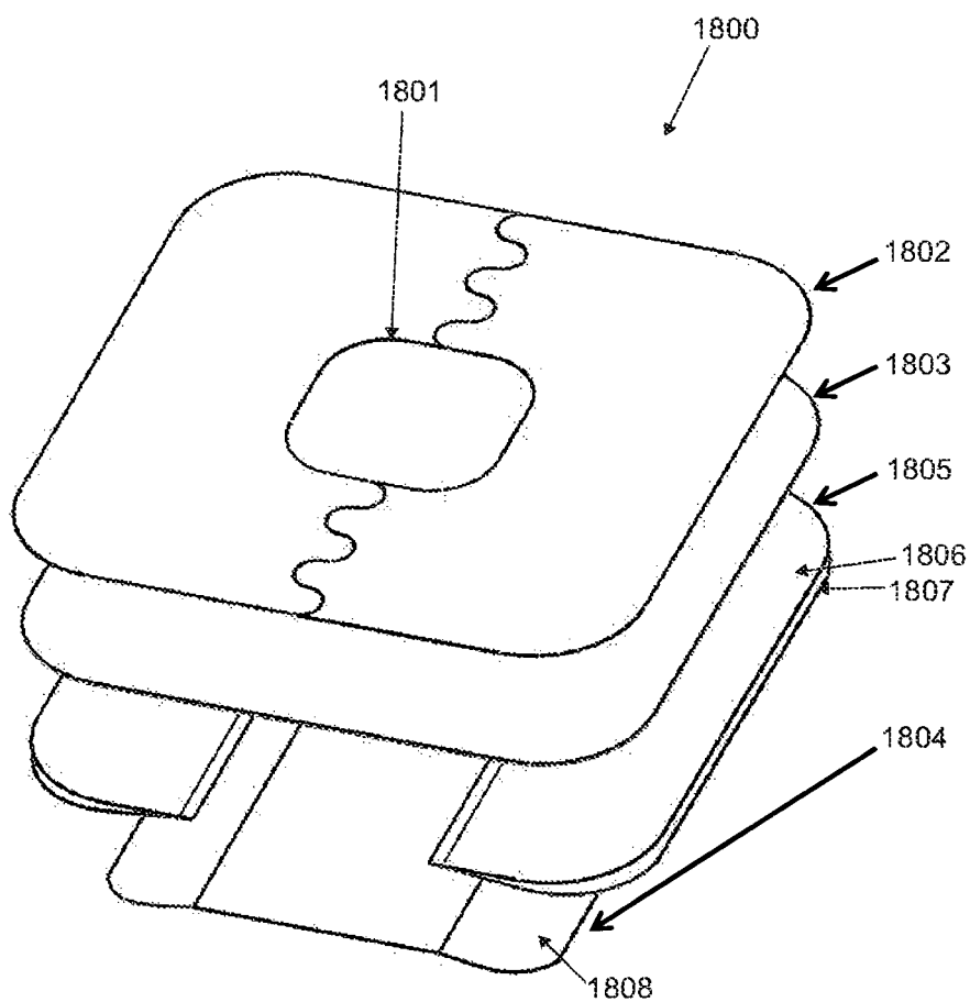
FIG. 18C
