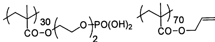
ポリマー（1）
