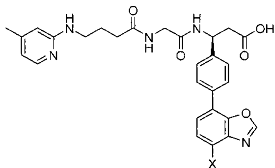
(Structure 12a),
