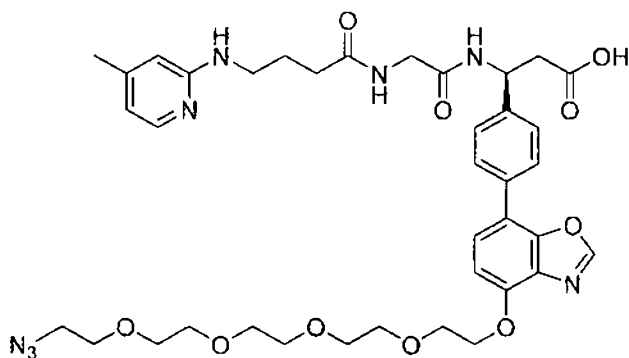
(Structure 12b)
