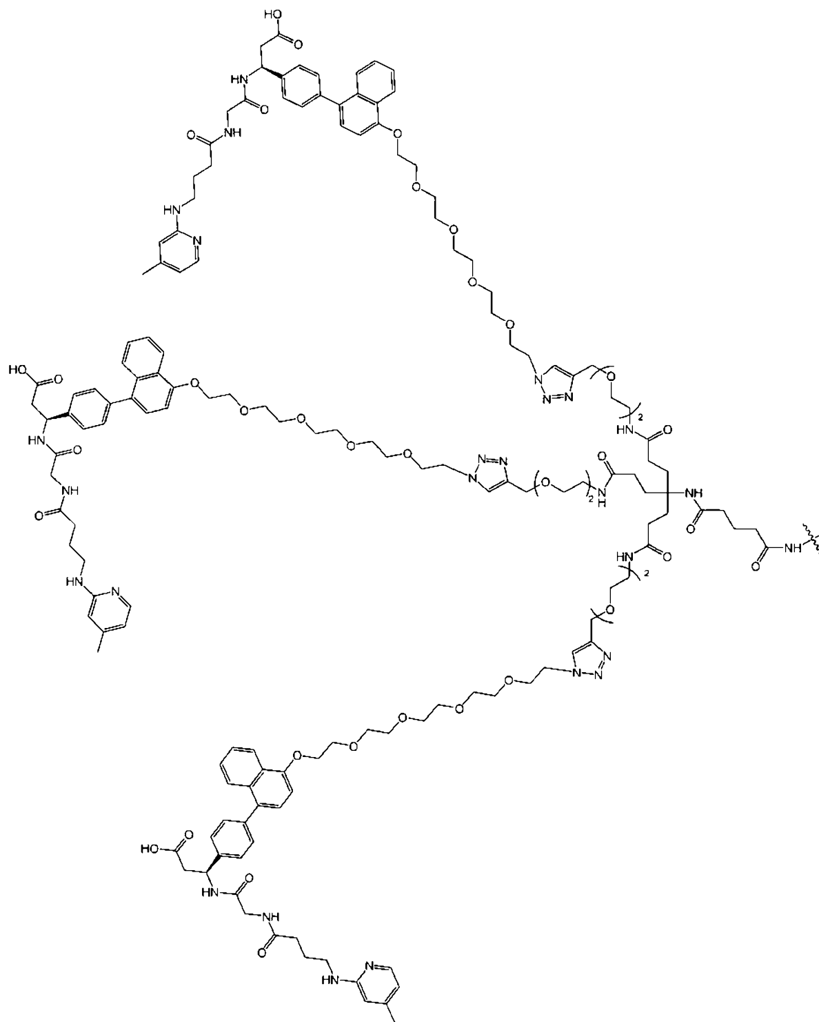
(Structure 701)
