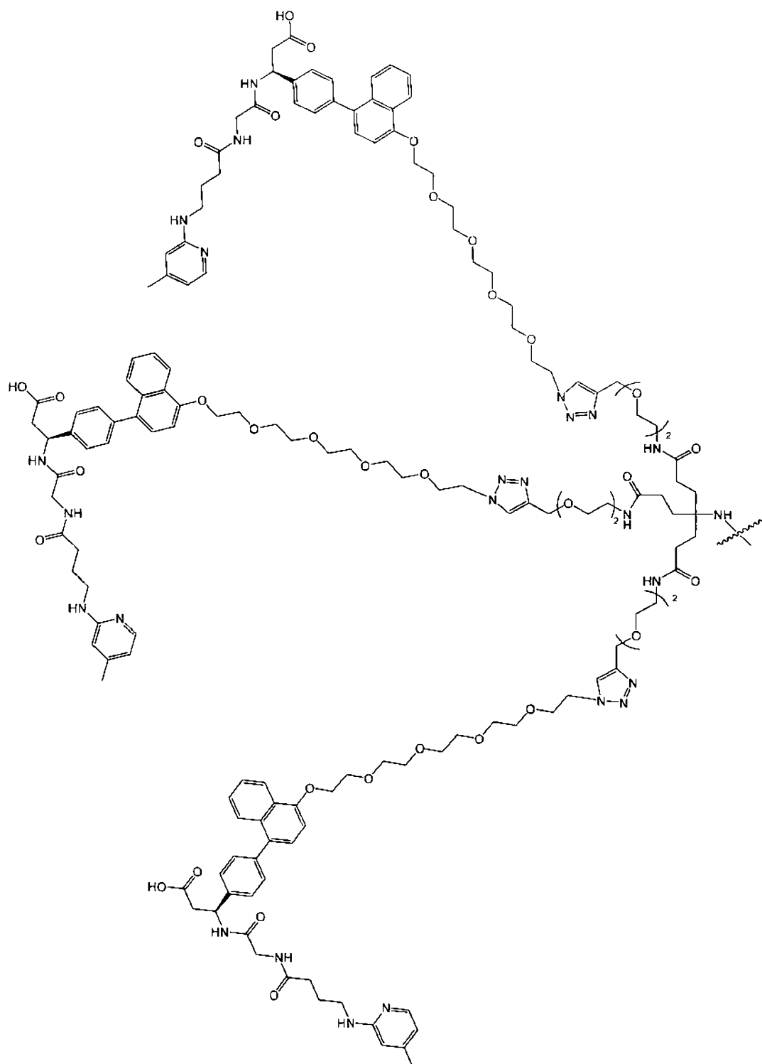
(Structure 701a)
