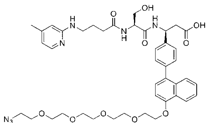
30b),
