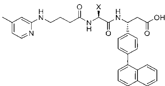
(Structure 9a),
