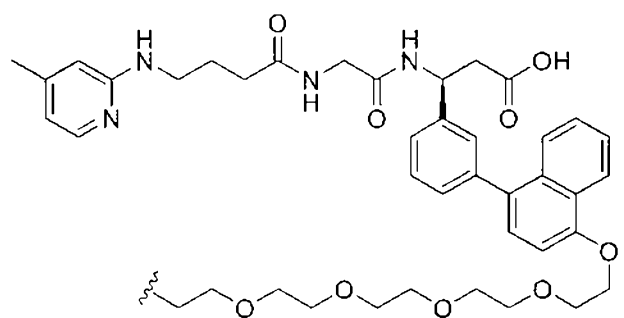
(Structure 20);
