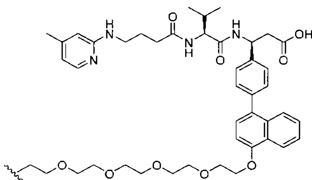
(Structure 23)
