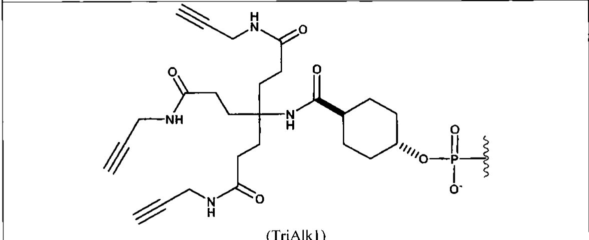
CC#CCNC(=O)CCC(CCC(=O)NCC#C)C(CCC(=O)NCC#C)C(=O)N[C@H]1CCCC[C@H]1OP(=O)([S-])C (TriAlk1)s
