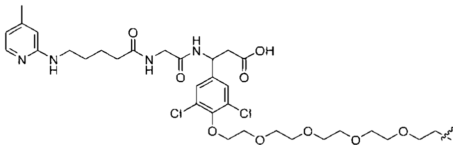
(Structure 5.1);
