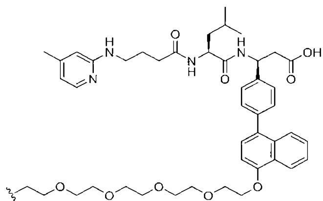
(Structure 34);
