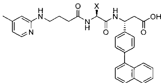
(Structure 9a),
