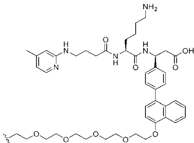
(Structure 33);
