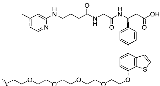
(Structure 17);
