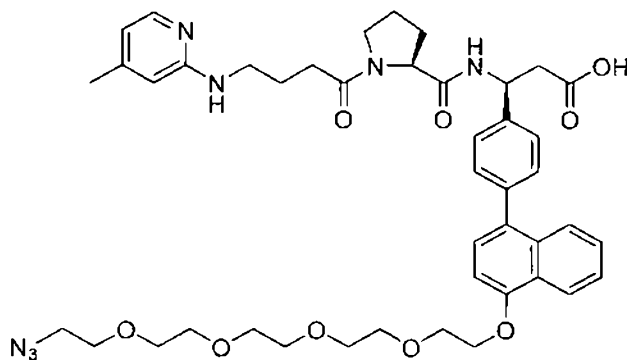
(Structure 11b)
