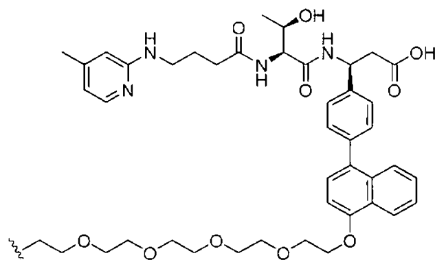
(Structure 35);
