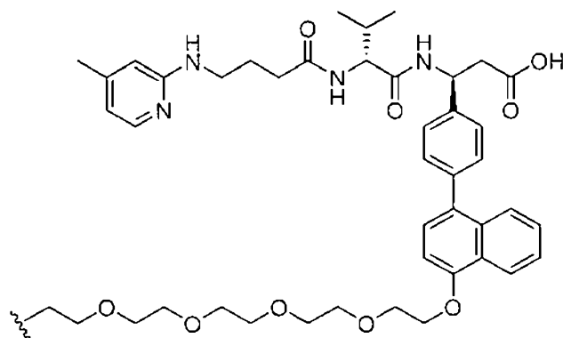
(Structure 37),
