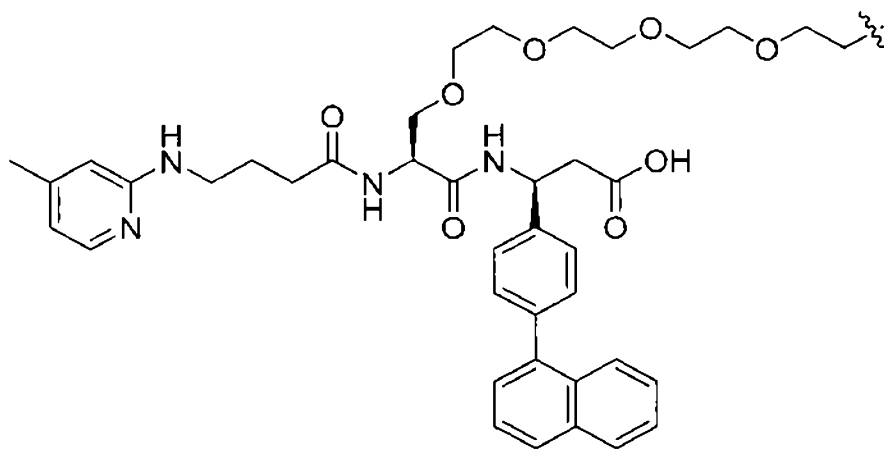
(Structure 1);
