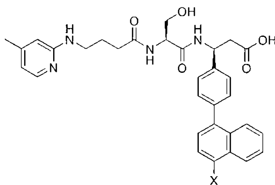
(Structure 31a),
