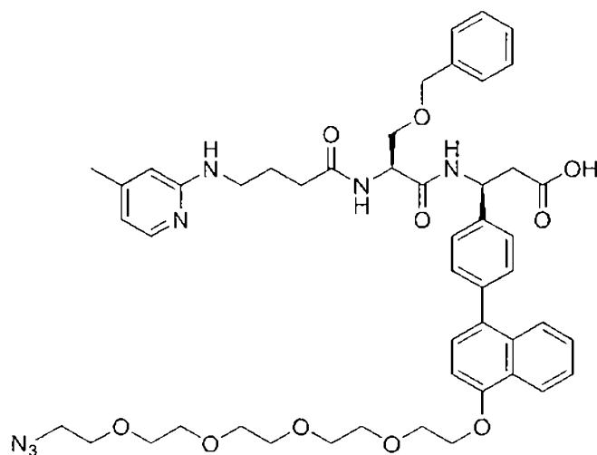
(Structure 25b),
