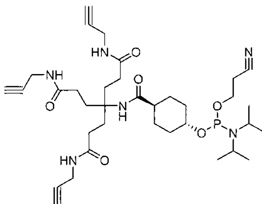
(Structure 400).
