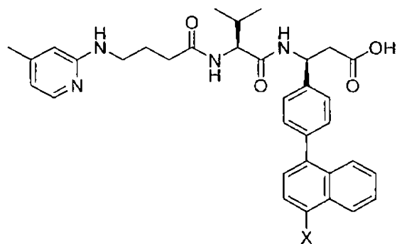
(Structure 23a),
