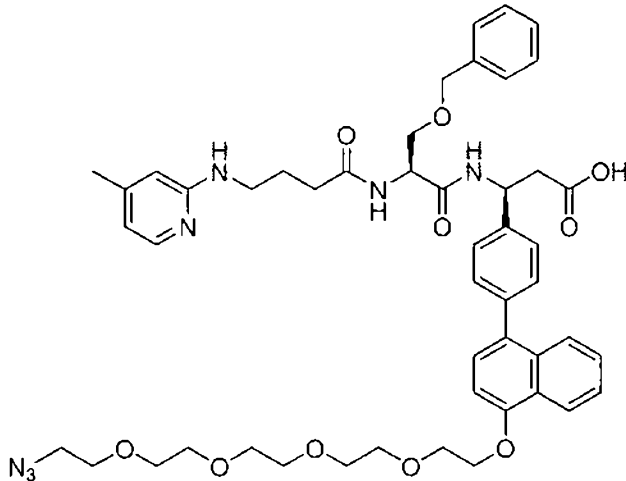
(Structure 25b)
