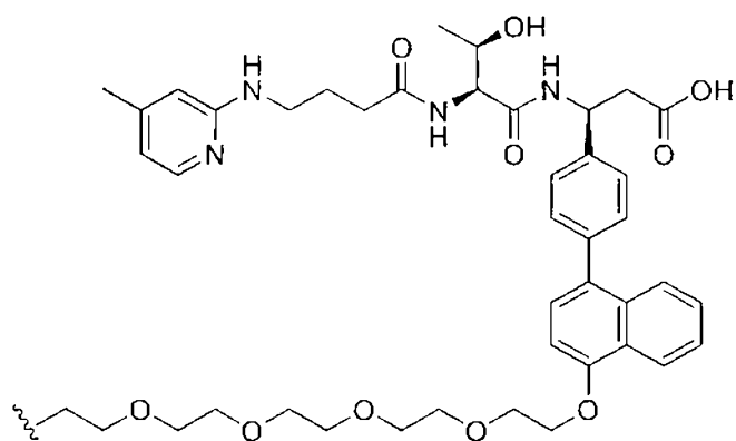
(Structure 35);
