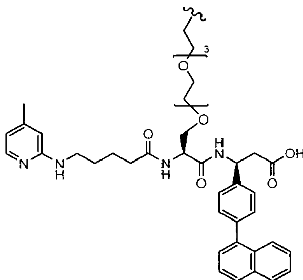
(Structure 1).
