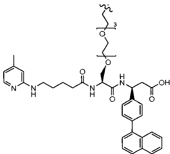
(Structure 1);
