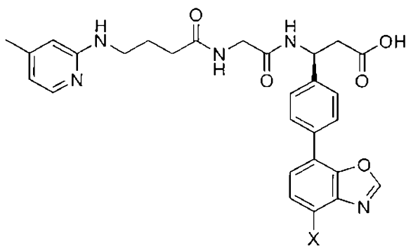
(Structure 12a),
