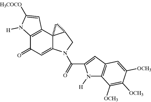
Duocarmycin SA
