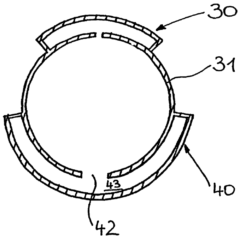
Fig. 6 B' - B'
