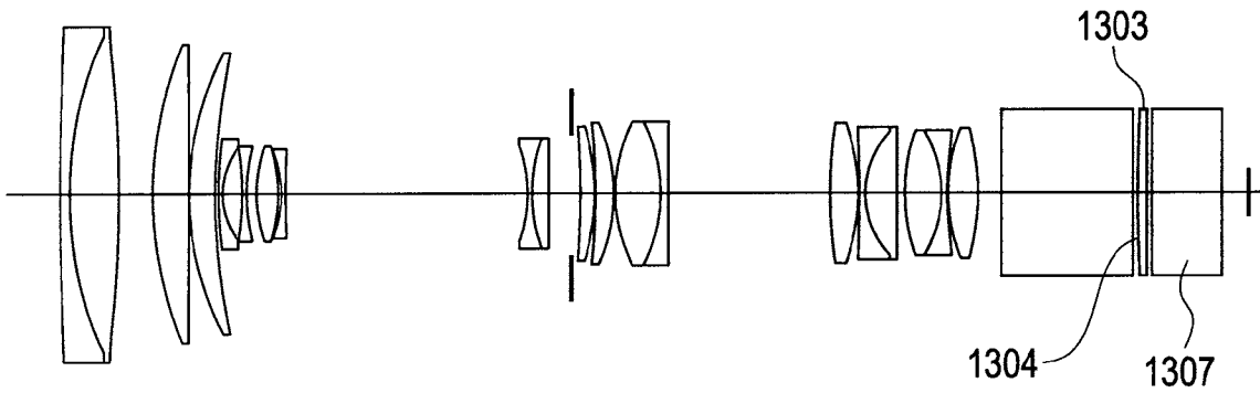
FIG. 15B
