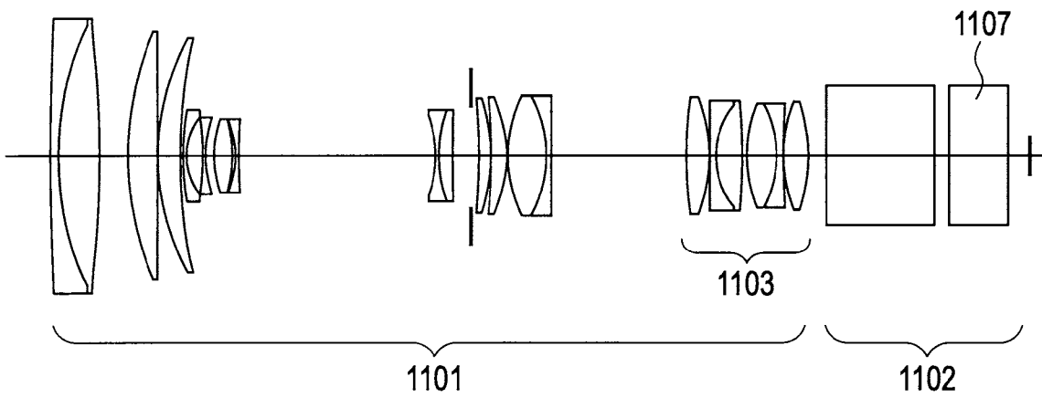
FIG. 13A
