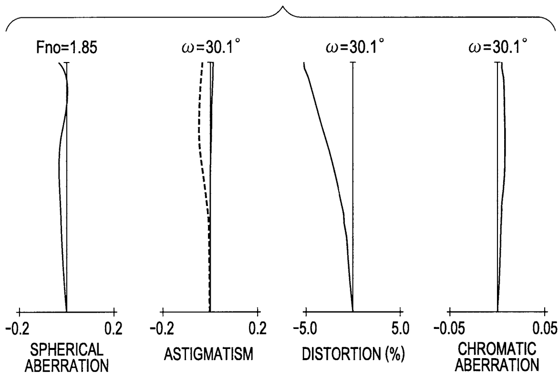
FIG. 14A
