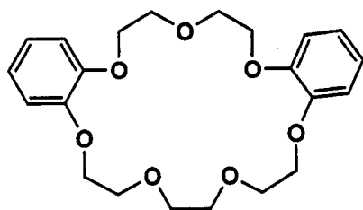
S-20
