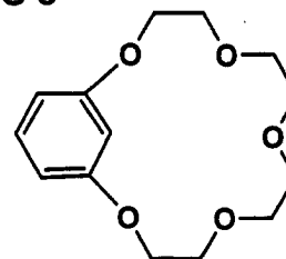
S-3
