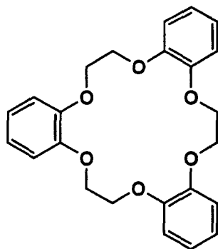
S-27
