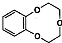
S-1
