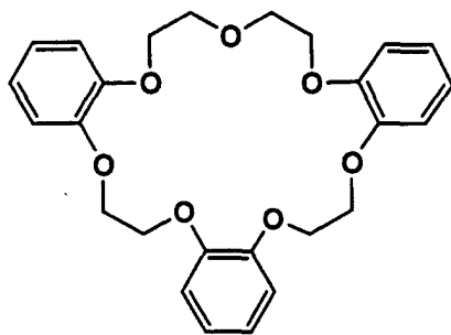
S-29
