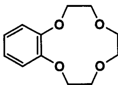
S-2
