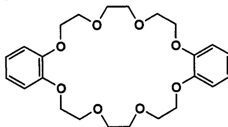
S-21
