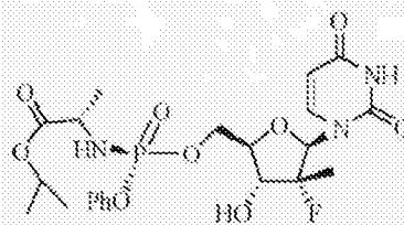
R p -4
