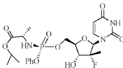
R P -4
