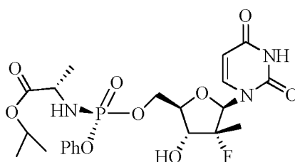
R_P - 4
