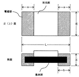
チップ抵抗 (10Ω~10MΩ) サイズ表 Type1 Type2
