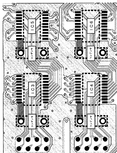
回路パターンの構成例の説明 2
