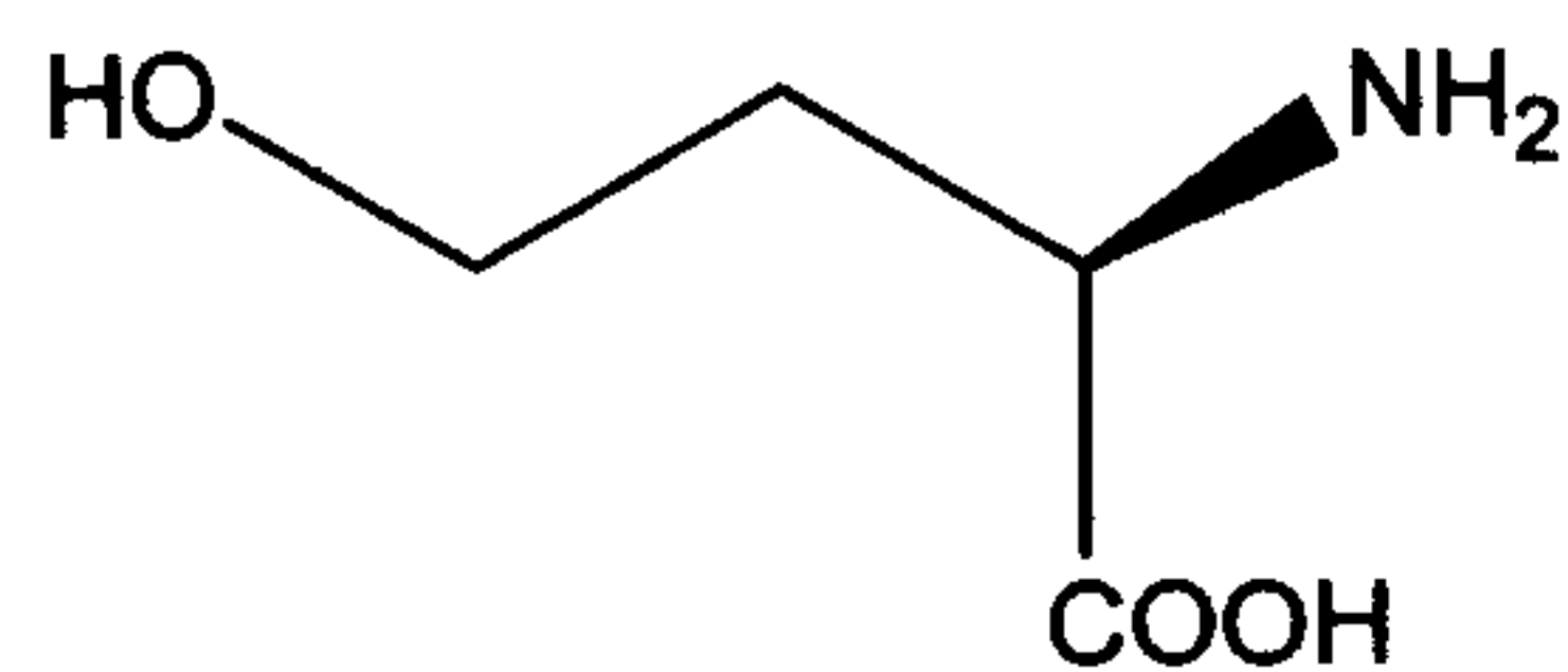
D-homoserine
