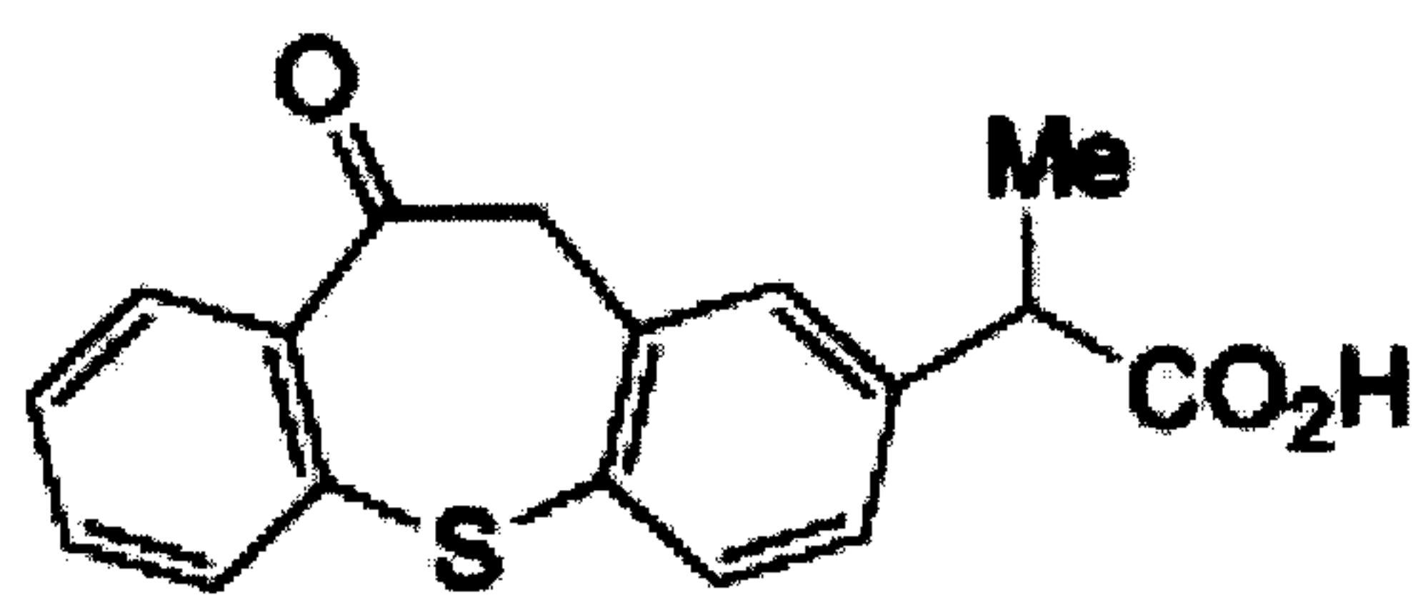
Zaltoprofen
