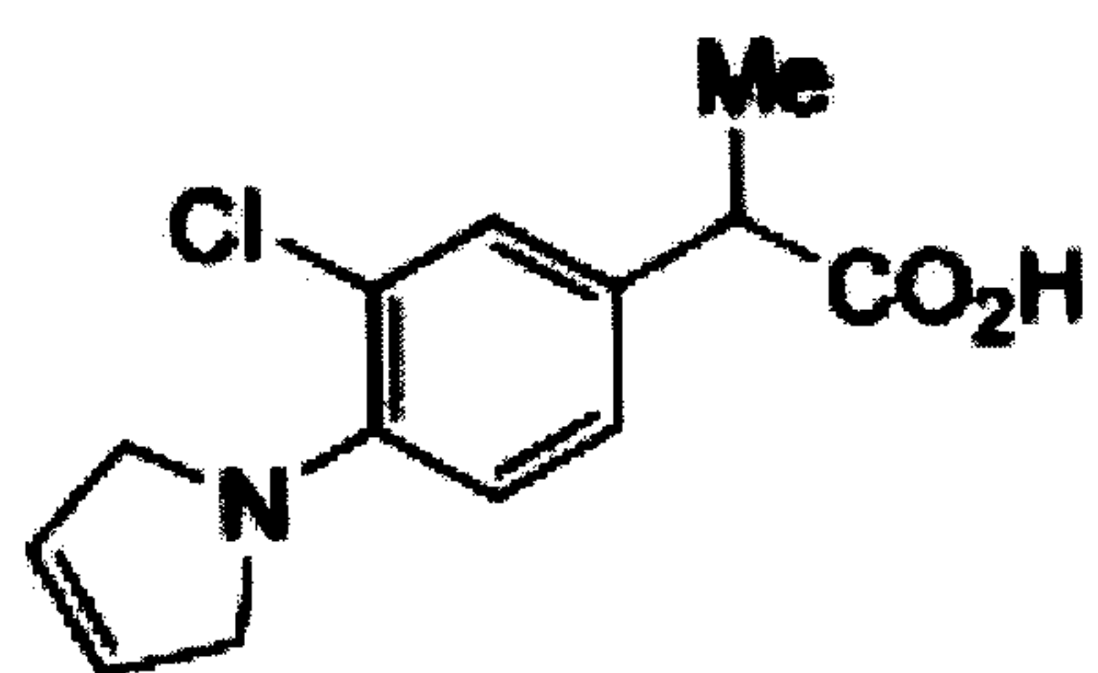
Pirprofen
