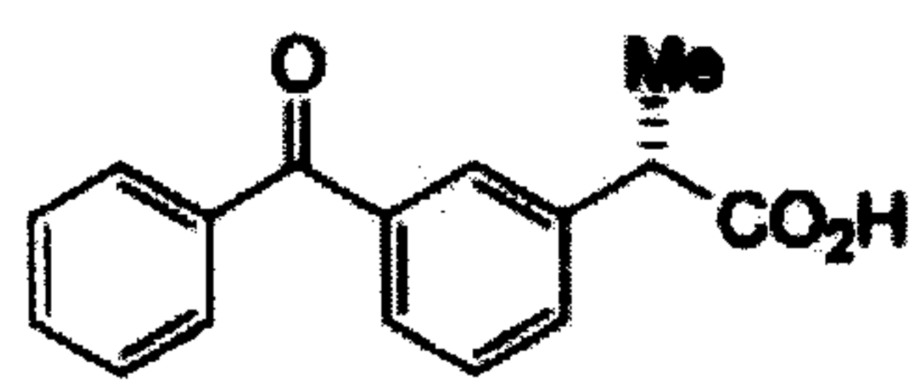
Dexketoprofen
