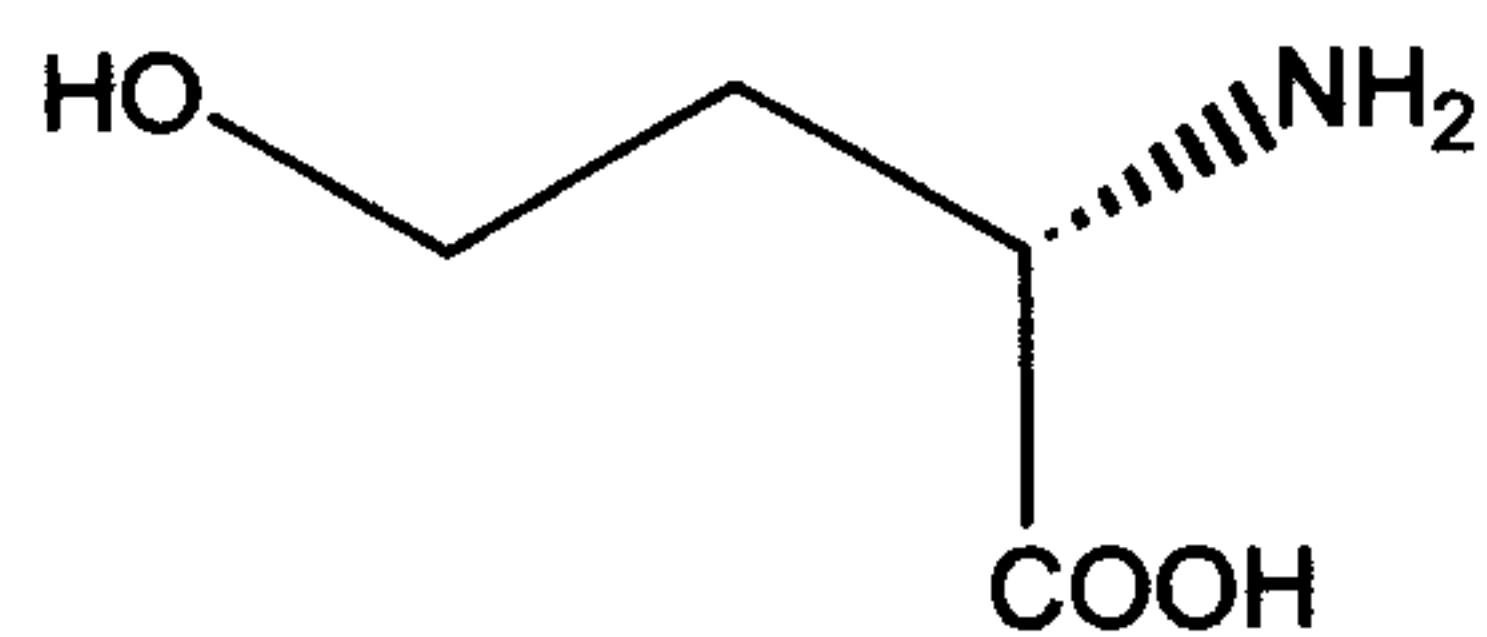
L-homoserine
