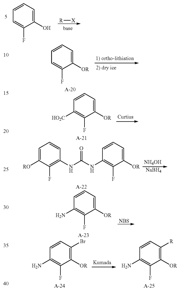
Scheme (IV)
