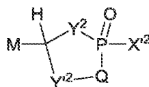
[0076] (IIa)
