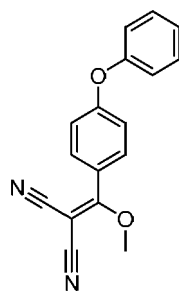
BG-3
