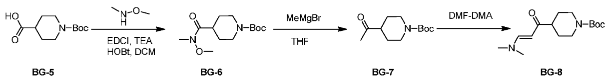
BG-5
