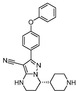
Formula 1e
