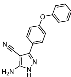
BG-4
